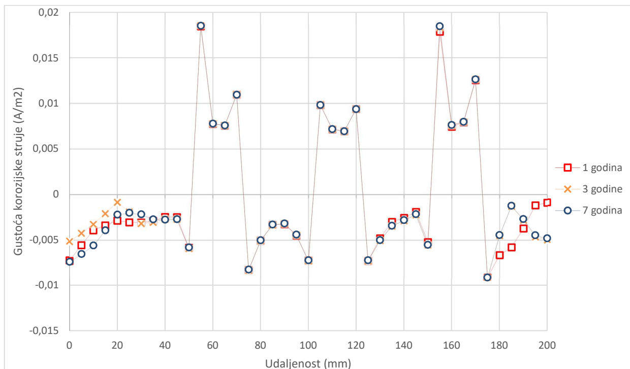
Slika 7.44. Graf raspodjele gustoće korozivne struje (A/m²) duž glavne armaturne šipke na modelu A2
