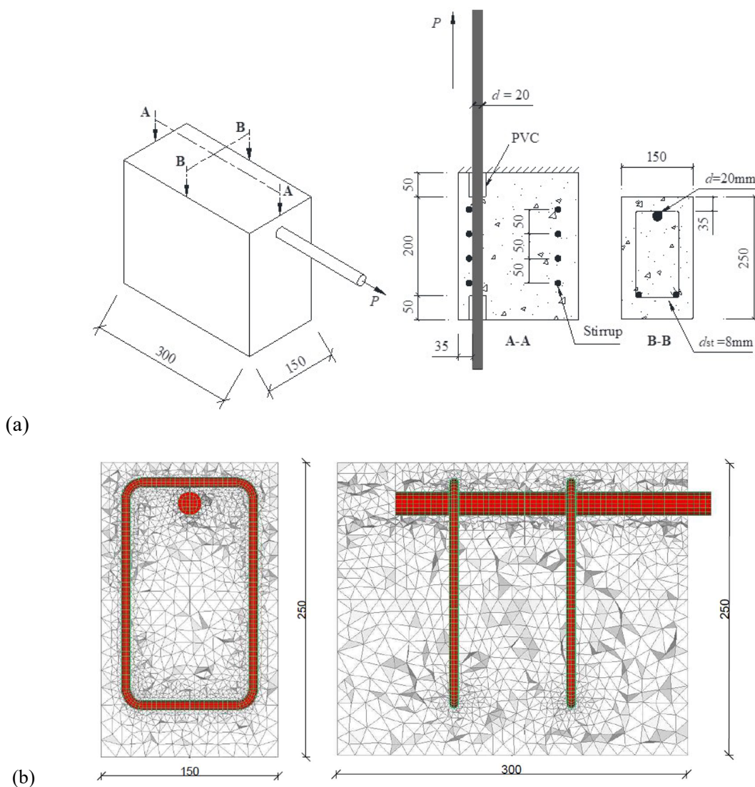
Slika 7.105. Prikaz geometrije uzorka: (a) skica eksperimentalnog uzorka [14] (b) prikaz numeričkog modela za ubrzanu koroziju
