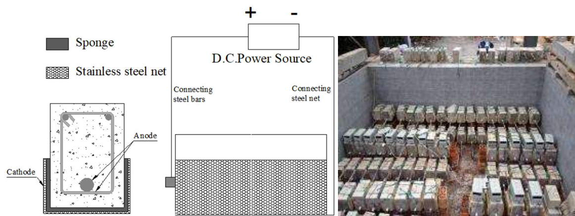
Slika 7.107. Ubrzana korozija: (a) šematski prikaz ubrzanе korozije; (b) uzorci uslijed ubrzanе korozije[14]
