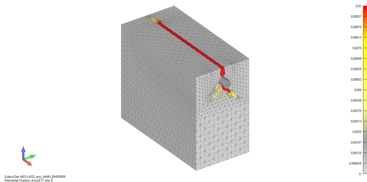
Slika 7.78. Prikaz oštećenja armiranobetonskog uzorka nakon provedenog pull-out testa na modelu B2 koji je prethodno bio izložen ubrzanjoj koroziji 8 dana (pogled-aksonometrija)
