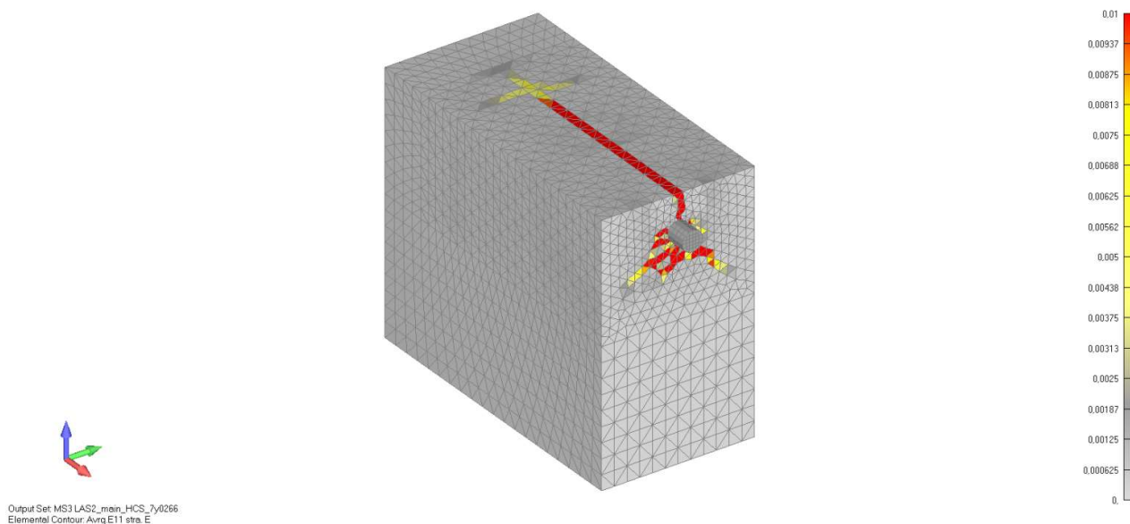
Slika 7.28 Prikaz oštećenja armiranobetonskog uzorka nakon provedenog pull-out testa na modelu A2 koji je prethodno bio izložen prirodnoj koroziji 7 godina dana (pogled-aksonometrija)
