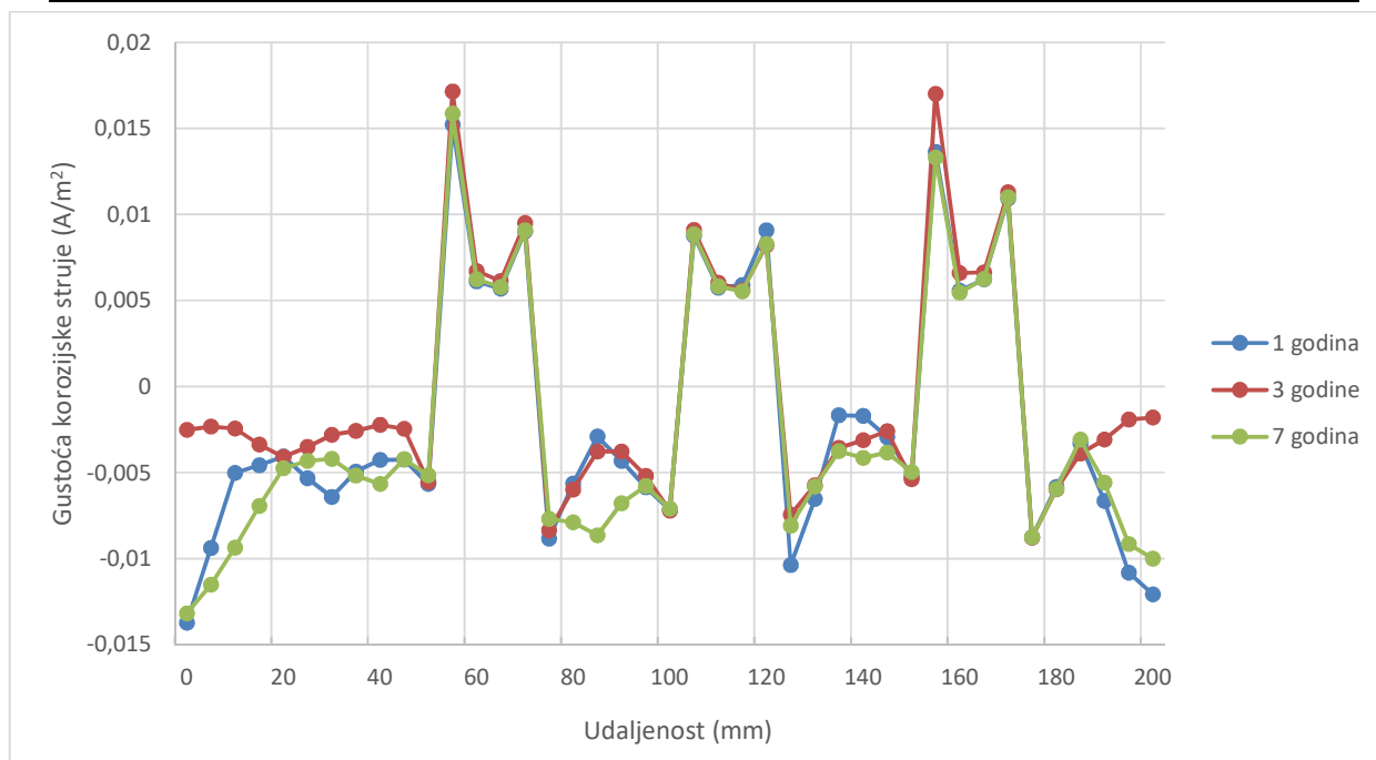
Slika 7.43. Graf raspodjele gustoće korozivne struje (A/m²) duž glavne armaturne šipke na modelu A1
