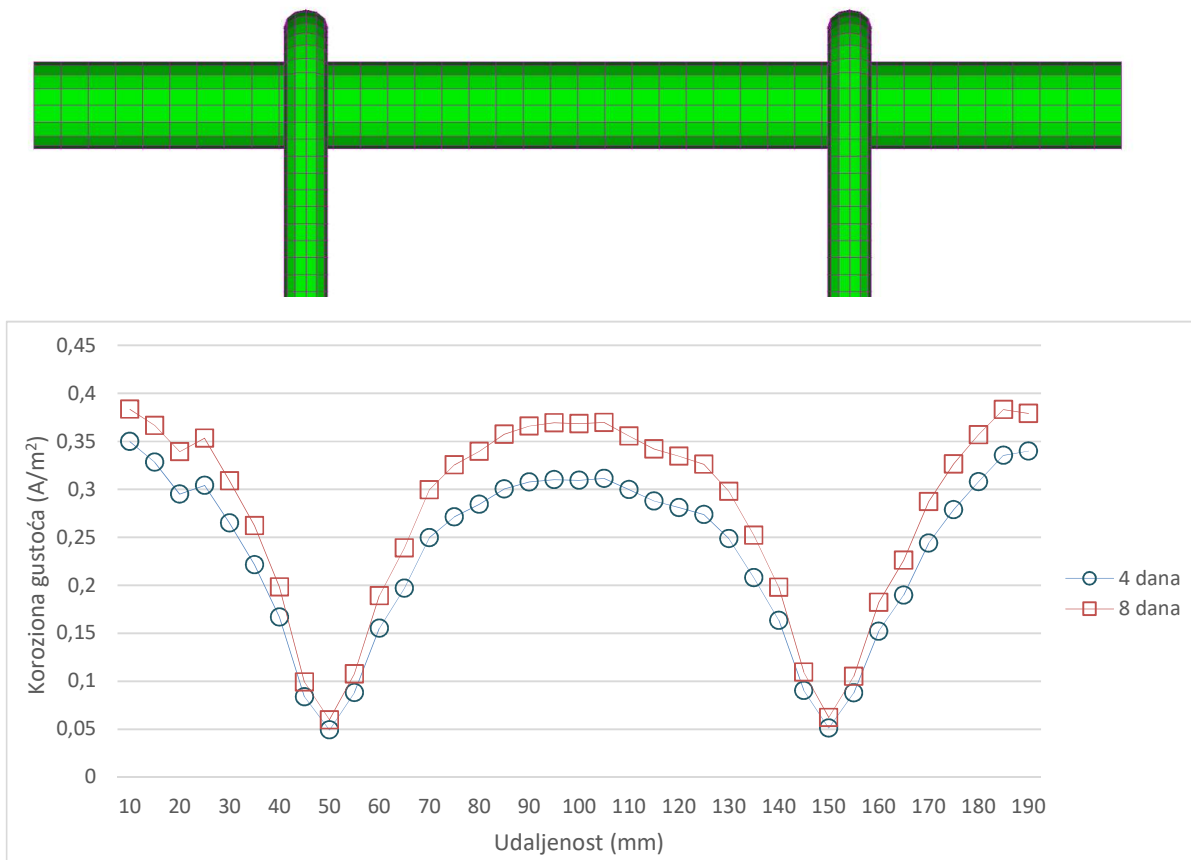
Slika 7.99. Gustoća korozivne struje na glavnoj šipci za ubranu koroziju nakon 4 i 8 dana
