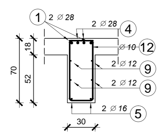
PRESJEK 3-3
