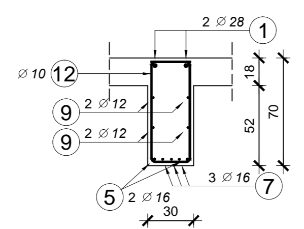
PRESJEK 2-2
