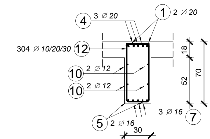
PRESJEK 1-1
