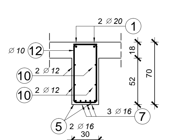
PRESJEK 2-2
