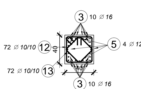
PRESJEK 4-4 40x40 (cm)
