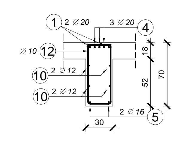
PRESJEK 3-3
