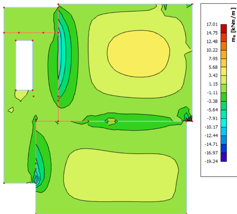
Slika 5.6 Prikaz momenata savijanja M_x GSU-1
