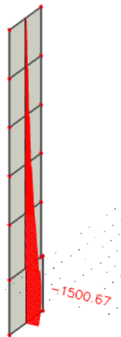
Slika 5.8. Uzdužna sila N od stalnog djelovanja
