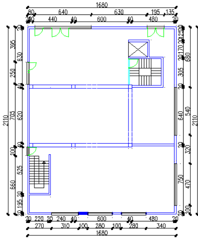
Slika 1.4. Tlocrt prizemlja
