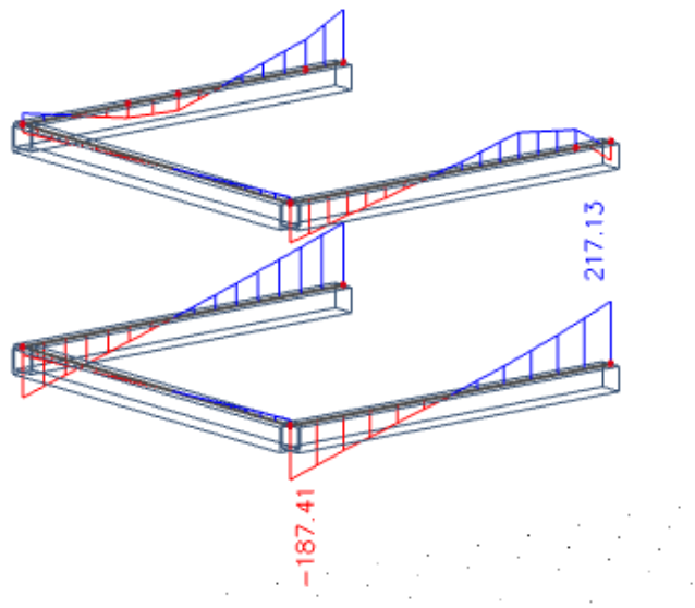
Slika 4.26. Maximalna poprečna sila V_z za kombinaciju 1,35G+1,5Q+1,5\cdot 0,6W za grede 40\times 40\text{cm}
