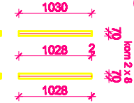
V4 70x70x3, l=832 mm, kom 2 x 8
