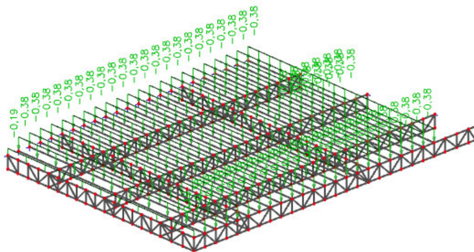
Slika 34: Prikaz raspodjele opterećenje snijegom-krov
