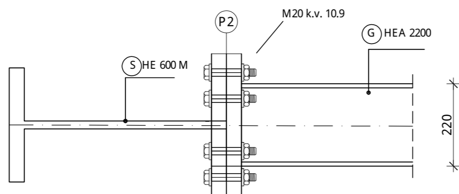
PRESJEK C-C
