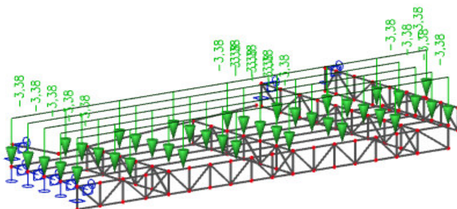
Slika 8: Prikaz raspodjele dodatnog stalnog opterećenje-galerija
