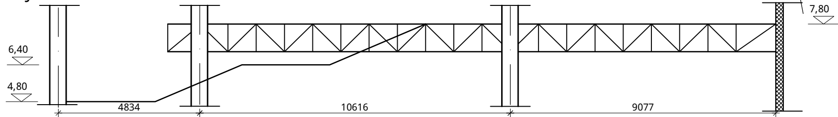
PRESJEK A - A
