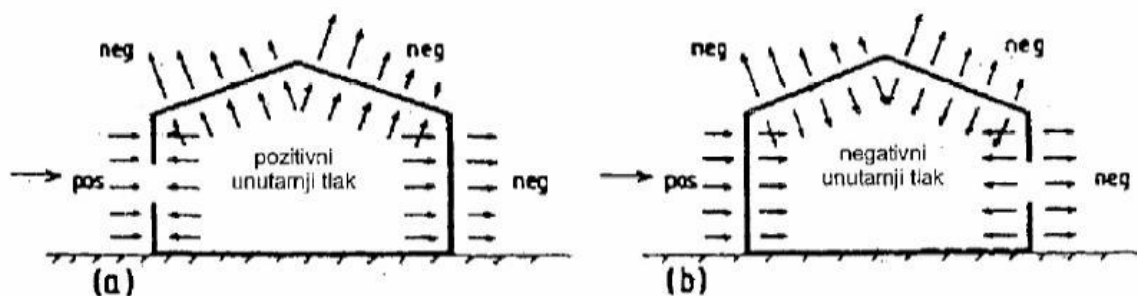
Slika 21: Pritisak vjetra
