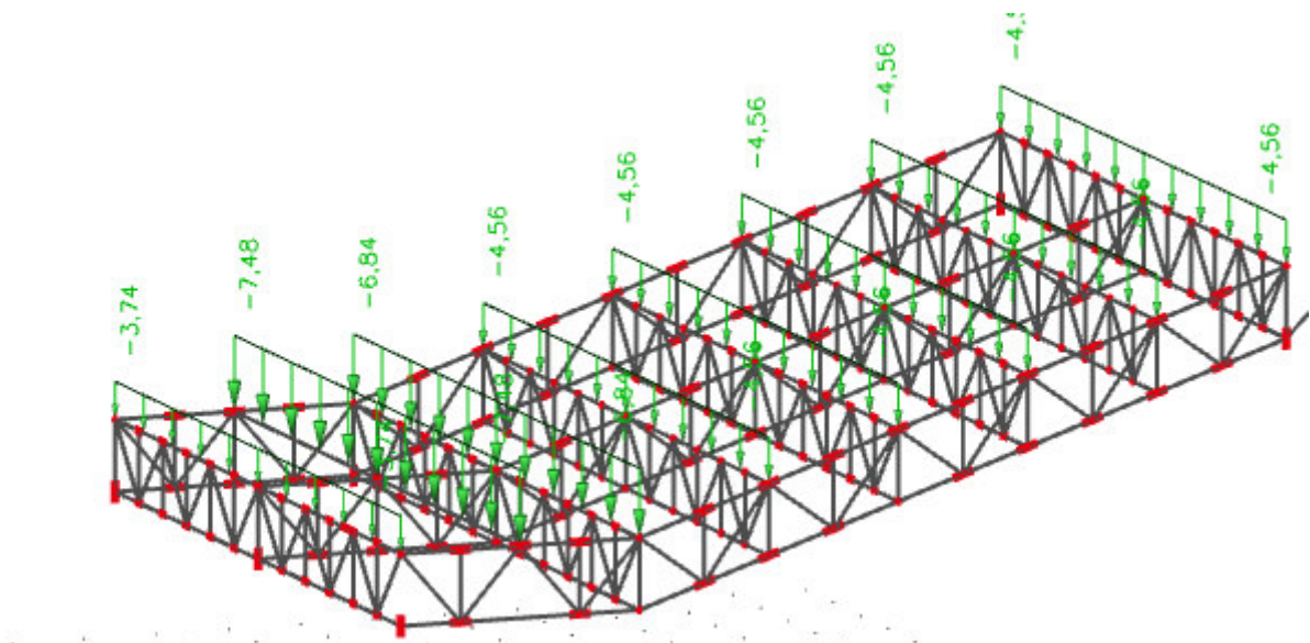
Slika 13: Prikaz raspodjele dodatnog stalnog opterećenja -amfiteatar
