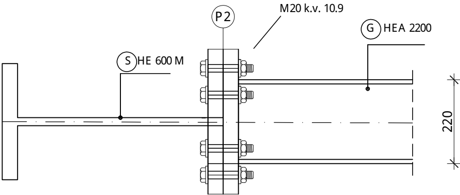
PRESJEK C-C
