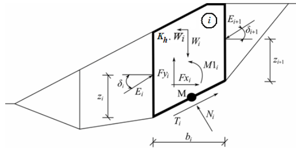
Slika 7.4 Analiza stabilnosti metodom blokova
