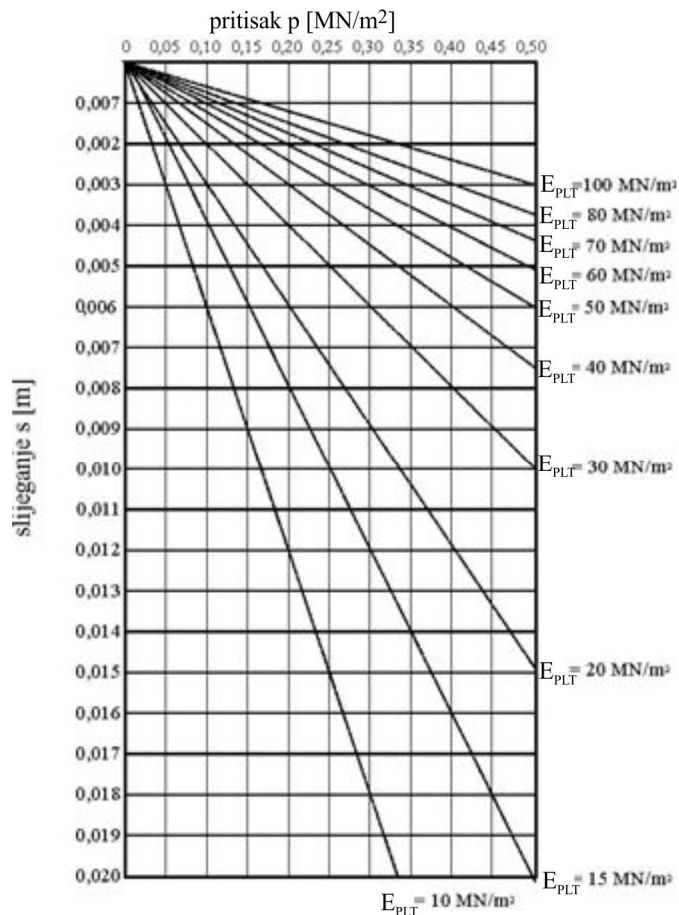
Slika 5.10 Obrazac za određivanje modula stišljivosti na terenu
