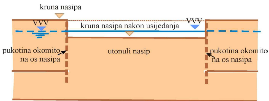
Slika 8.13 Usjedanje nasipa
