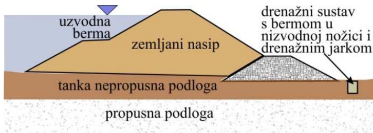
Slika 6.21 Hidrotehnički nasip na tankoj nepropusnoj podlozi - povratna erozija
