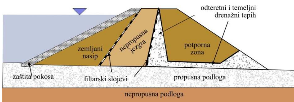
Slika 6.26 Višestruko zonirani nasip na propusnoj podlozi
