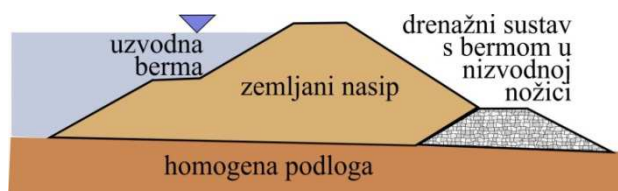
Slika 6.17 Homogeni hidrotehnički nasip s bermom i drenom u nožici na homogenoj podlozi
