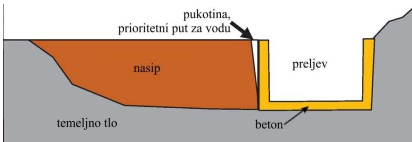
Slika 8.30 Pukotina uz betonski zid
