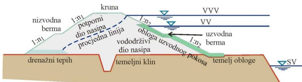
Slika 6.4 Hidrotehnički nasip s bitnim dijelovima
