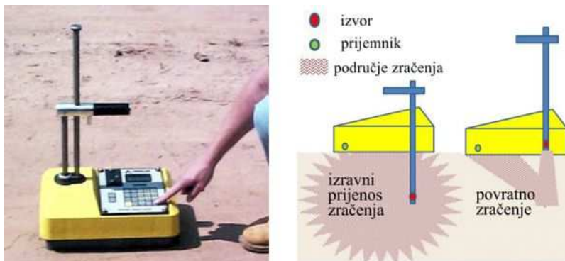
Slika 5.2 Mjerenje gustoće tla nuklearnim denzimetrima
