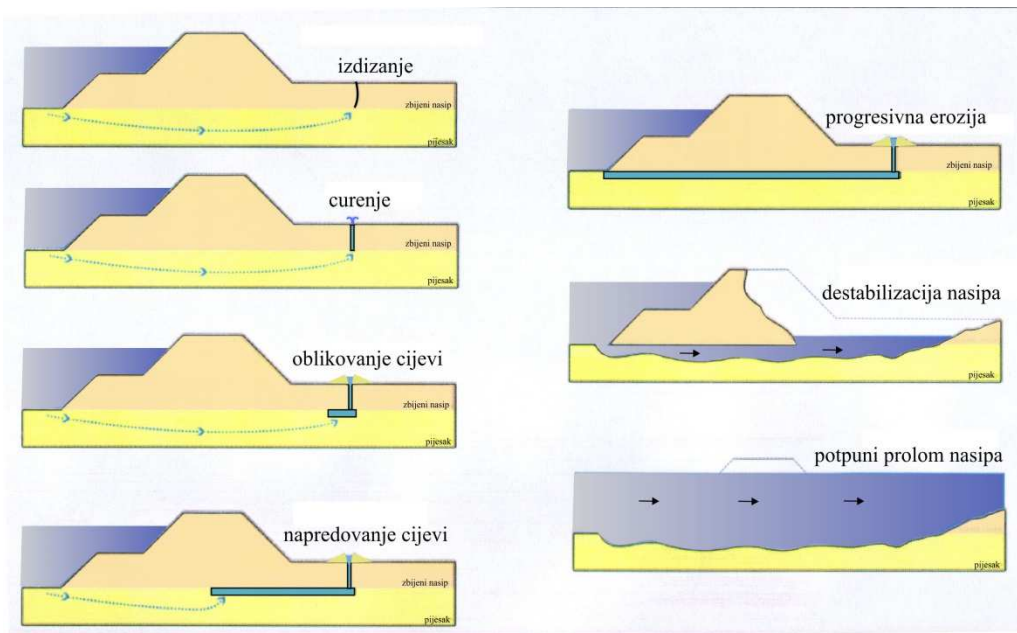
Slika 8.38 Proces povratne erozije kroz propusnu podlogu (Van Beek i dr. 2010.)
