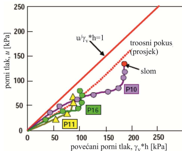
Slika 4.6 Zmjerene vrijednosti povećanih pornih tlakova tijekom gradnje nasipa
