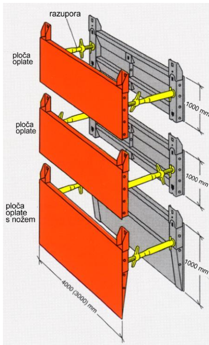
Slika 8.19 Sustav oplata za iskop kanala s pločama
