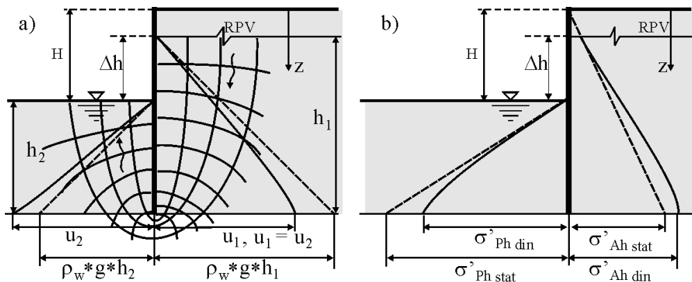
Slika 2.37 Dijagram hidrodinamičkog tlaka u usporedbi s hidrostatičkim a) i njegov utjecaj na promjenu bočnih efektivnih napreznja b)
