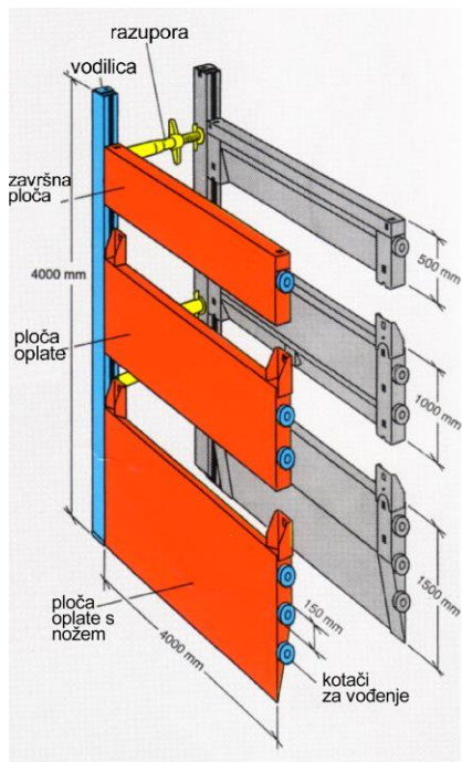
Slika 8.20 Sustav oplata s pločama i vodilicama
