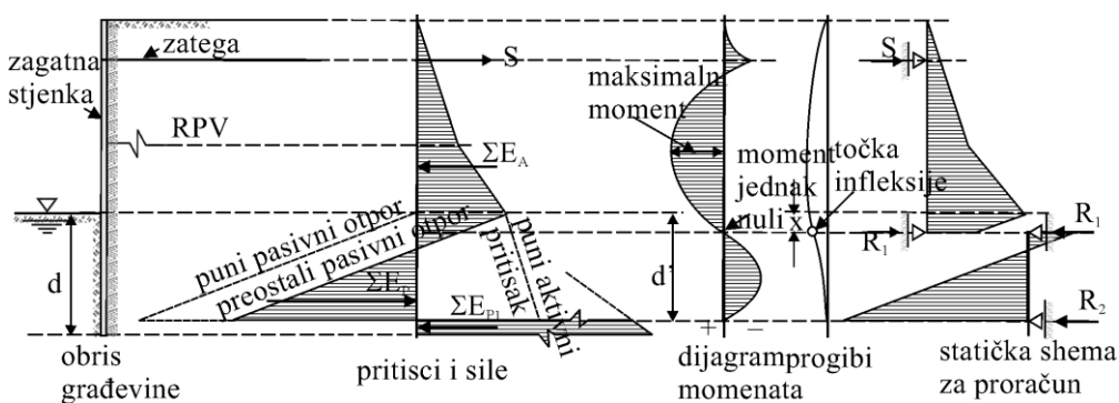
Slika 5.36 Usidrena zagatna stijenka, upeta na donjem kraju (s rješenjem metodom ekvivalentne grede)
