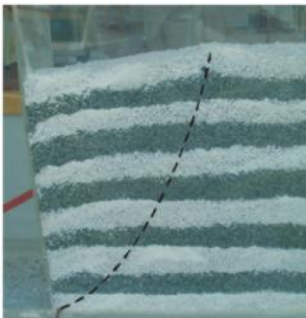
Slika 2.12 Laboratorijski model s rekonstruiranom kliznom plohom pri zaokretu podupore oko točke B, aktivno stanje (model autora)
