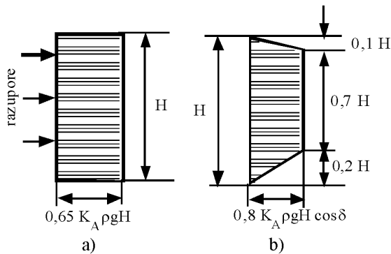
Slika 5.4 Raspodjela pritisa na podgradu u pijescima (Dismuke, 1991.)
