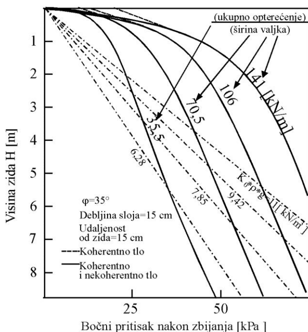
Slika 3.8 Primjer odnosa tlaka mirovanja i pritiska valjka pri zbijanju nasipa iza potpornog zida (Duncan i sur., 1991.)
