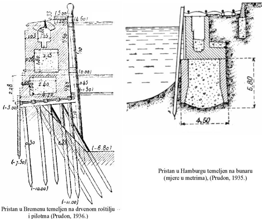
Slika 3.2 Masivni, gravitacijski potporni zidovi na dubokim temeljima
