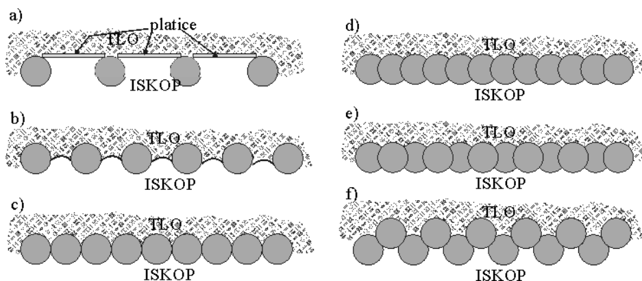
Slika 5.46 Mogući raspored pilota pri njihovom korištenju kao zagatne stijenske
