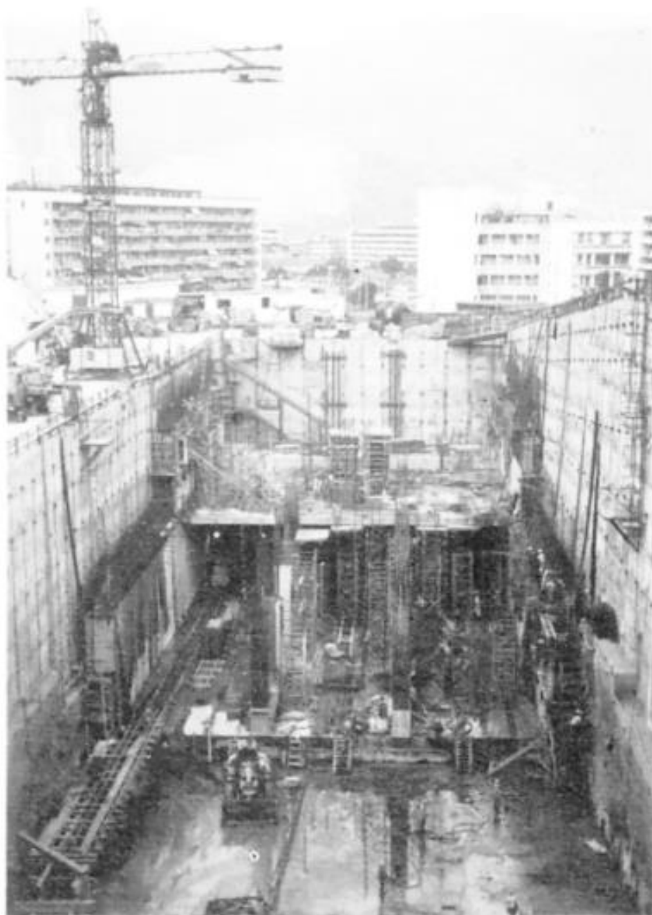
Slika 1.5 Građevna jama podzemne željeznice u Hong-Kongu (Gardey, 1978.)
