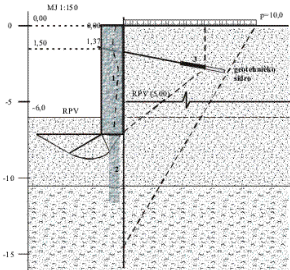
Slika 1.11 Primjena suvremene tehnologije: 1 mlezno-injektirani stupnjaci \Phi=150 cm s preklapom od 20 cm; 2 mlezno-injektirane lamele d=40 cm; 3 sidro, (Keller, 2003.),
