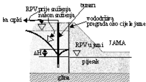
Slika 8.61 Smanjenje hidrostatičkog pritiska na vododrživu zavjesu pomoću bunara
