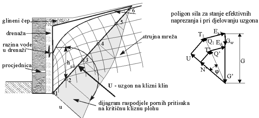
Slika 2.38 Utjecaj hidrodinamičkog pritiska na kritični klizni klin pri naglom pljusk
