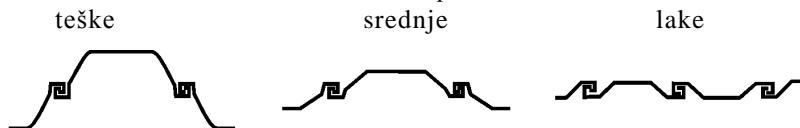
Slika 5.21 b: tip Larsen
