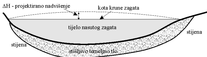
Slika 6.7 Nadvišenje zagata
