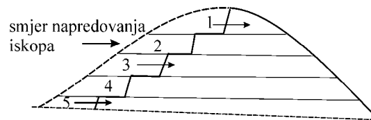
Slika 8.32 Iskop u terasama po cijeloj dužini poteza
