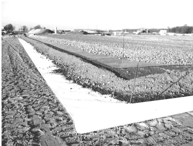
Slika 11.15 Ojačanje posteljice i nasipa geomrežom i geotekstilom
