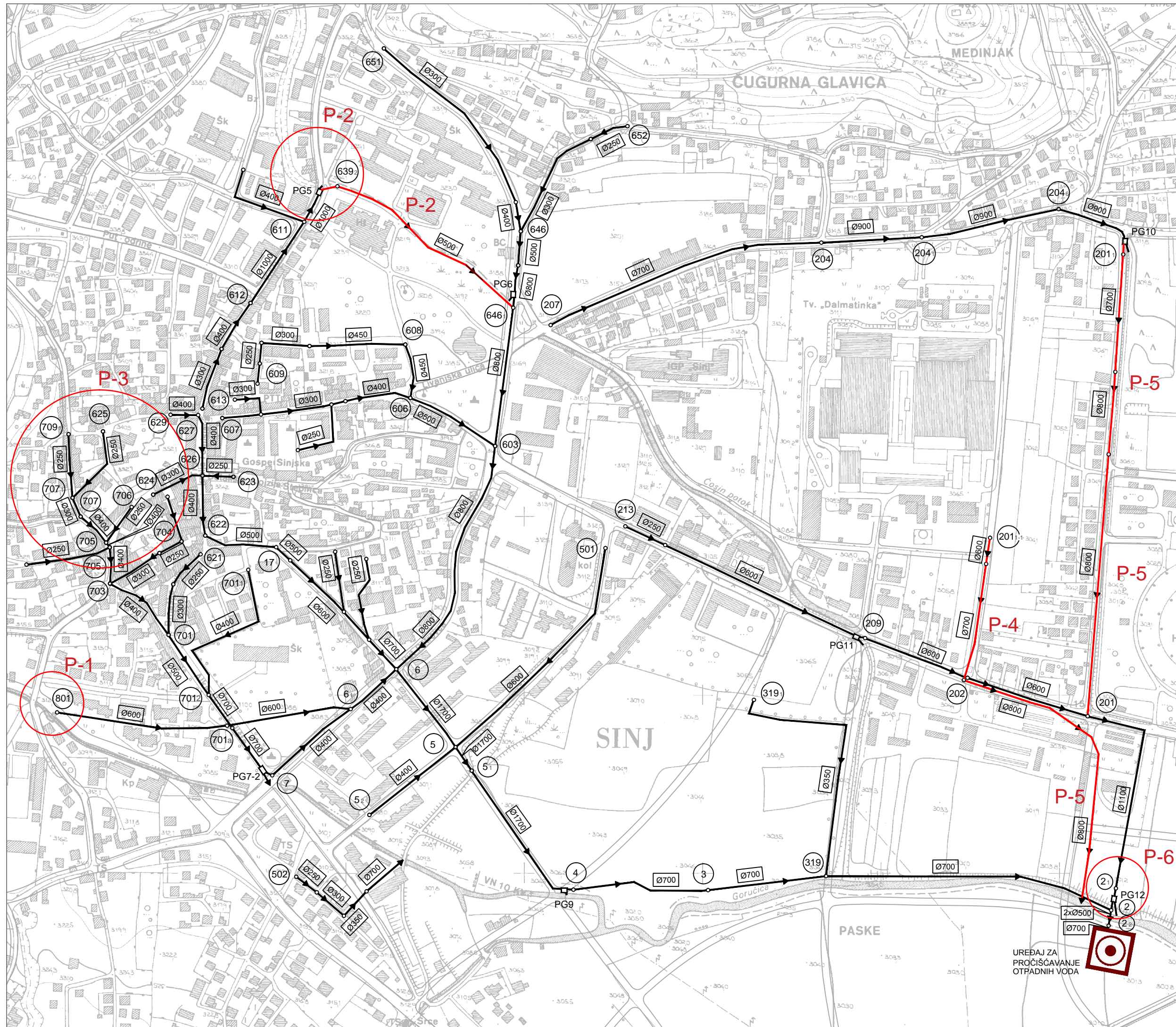
SITUACIJA PROBLEMI POSTOJEĆEG STANJA MJ. 1:2500 LEGENDA: POSTOJEĆA MJEŠOVITA KANALIZACIJA POSTOJEĆA PRELJEVNA GRAĐEVINA UREĐAJ ZA PROČIŠĆAVANJE OTPADNIH VODA OZNAKA REVIZIJSKOG OKNA
