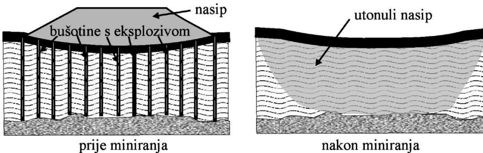
Slika 9.40 Zamjena tla miniranjem na trasi buduće prometnice
