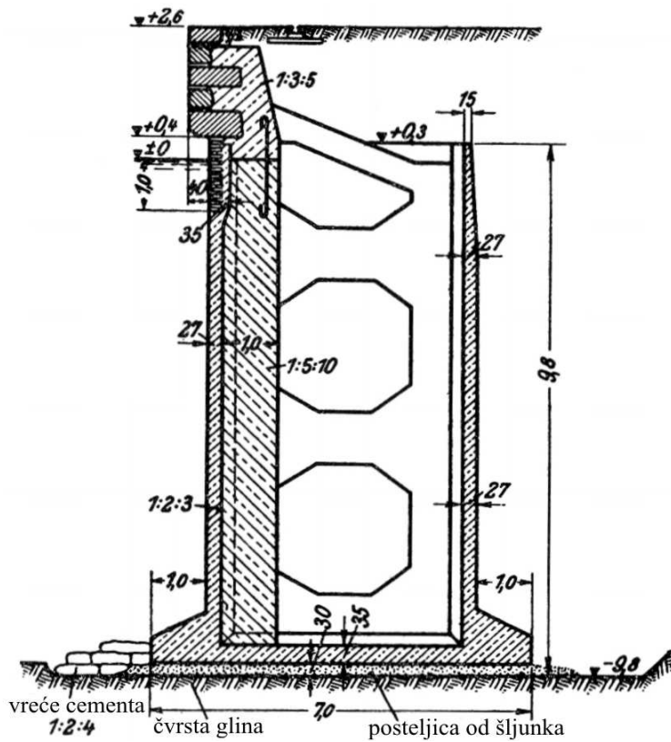
Slika 7.28 Obalni zid u Kölnu, Njemačka (Press, 1962.)
