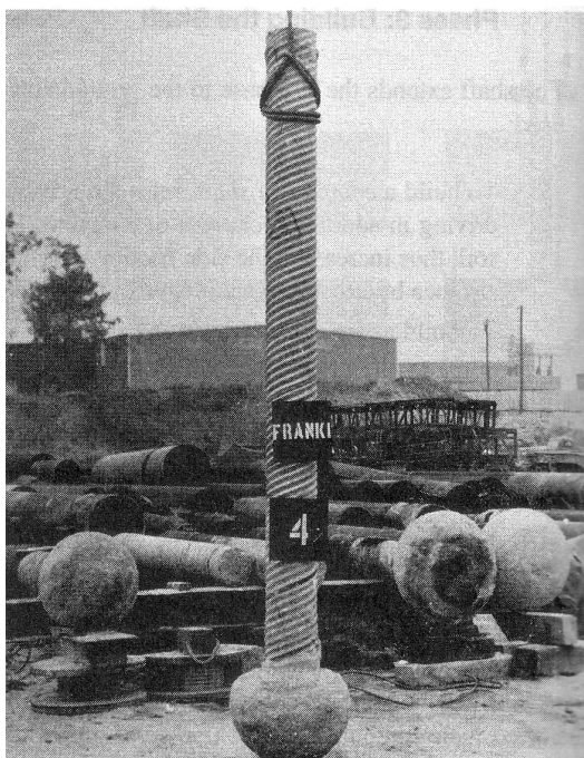
Slika 5.83 Pilot s glavom proširenom mlaznim injektiranjem (Coduto 2001.)
