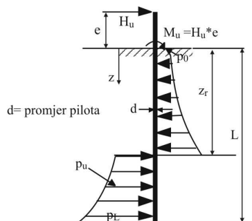
Slika 5.23 Skica raspodjele otpora tla duž pilota potrebna za proračun granične vrijednosti sile H=H_u (Poulos & Davis 1980.)]
