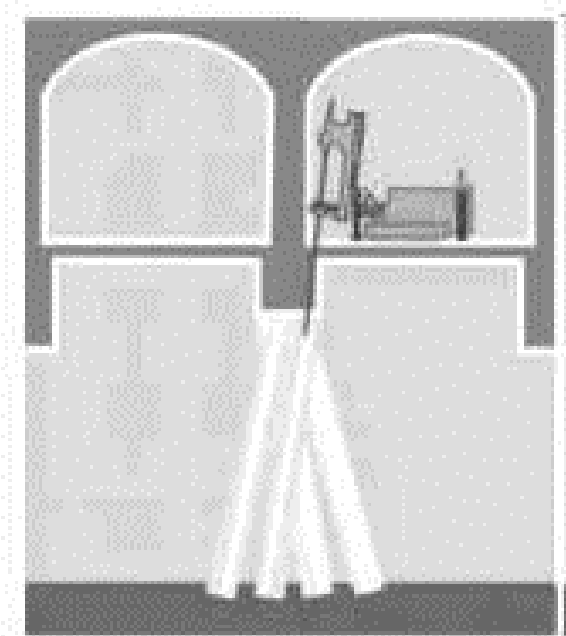
Slika 8.28 Produbljenje temelja do dobro nosivog sloja
