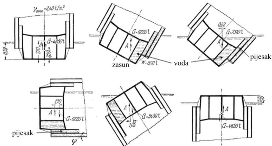
Slika 7.22 Potapanje plivajućeg sanduka okretanjem za 180°
