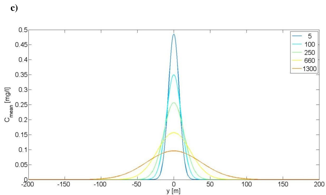
Slika 2.12 Prikaz srednje vrijednosti koncentracije ukupnog fosfora na ušću Jadra: a) u glavnom prozoru; b) na pozadinskoj mapi; c) za presjeke na različitim udaljenostima od ušća za minimalni ljetni protok iz 2017. godine
