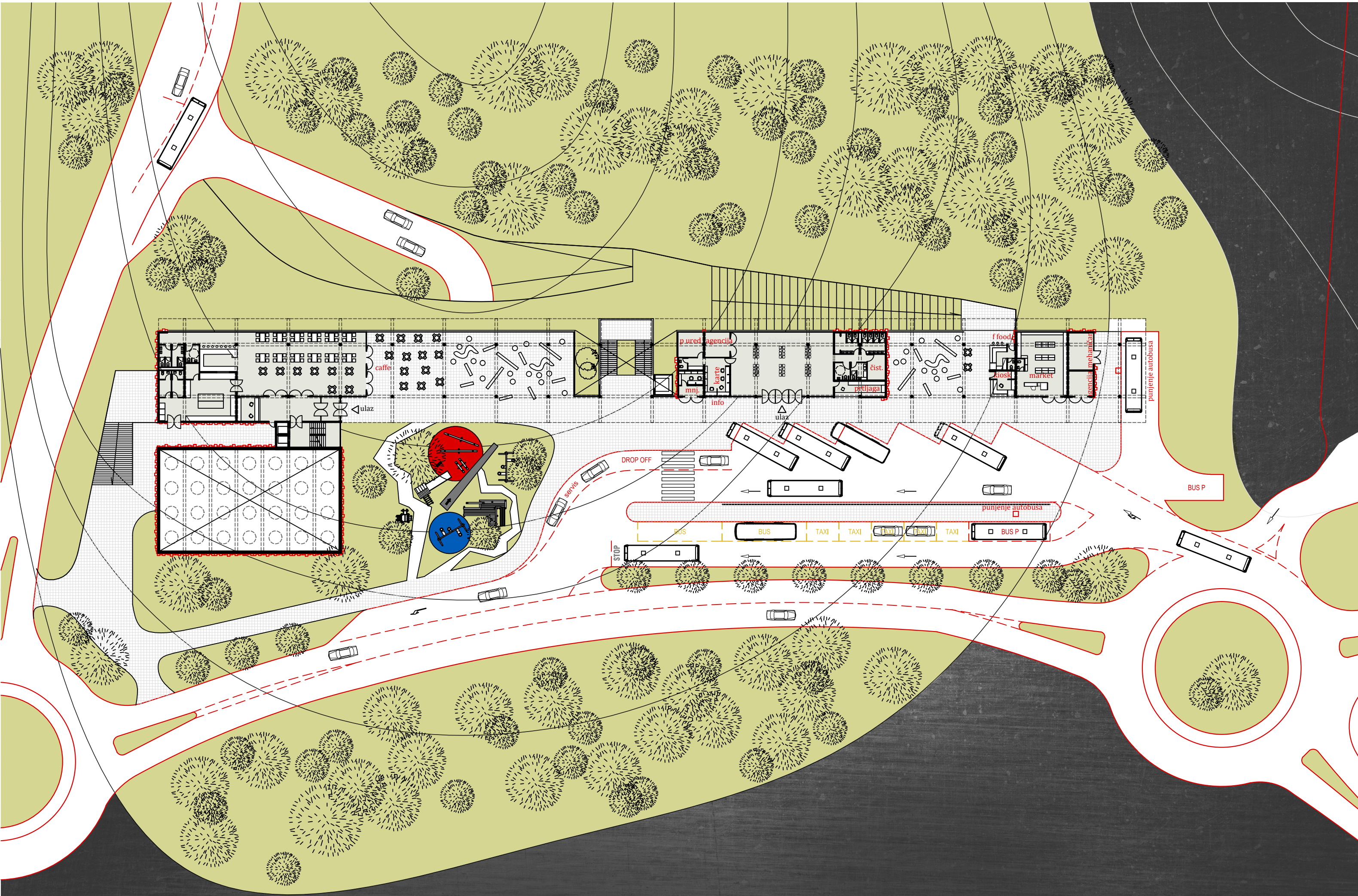
_tlocrt prizemlje
