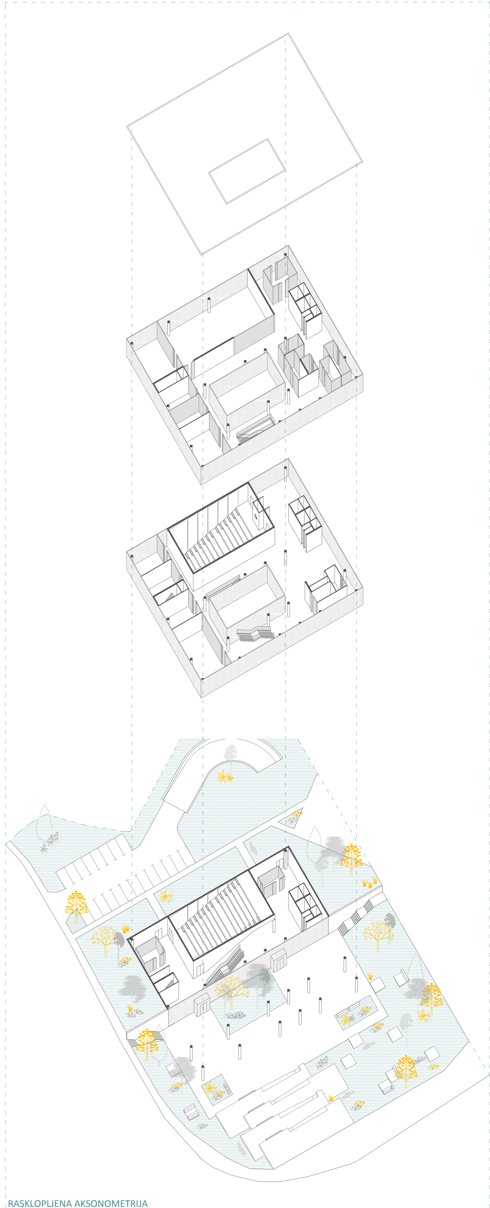
RASKLOPLJENA AKSONOMETRIJA
