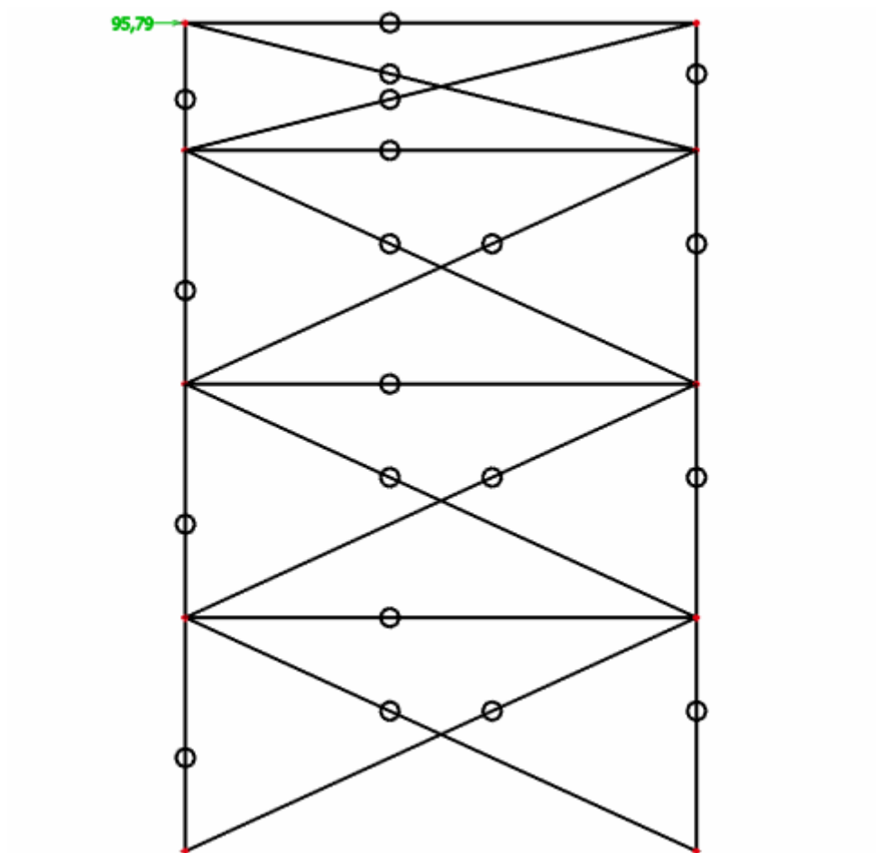
Slika 5.3. Raspored bočnih spregova i opterećenje
