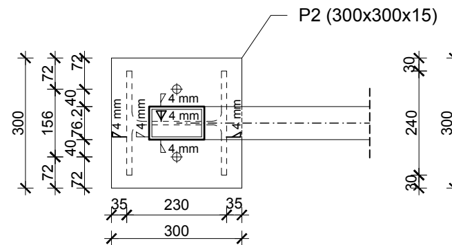
Presjek 2-2
