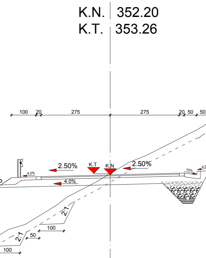
PROFIL 14 ST. 0+390.00
