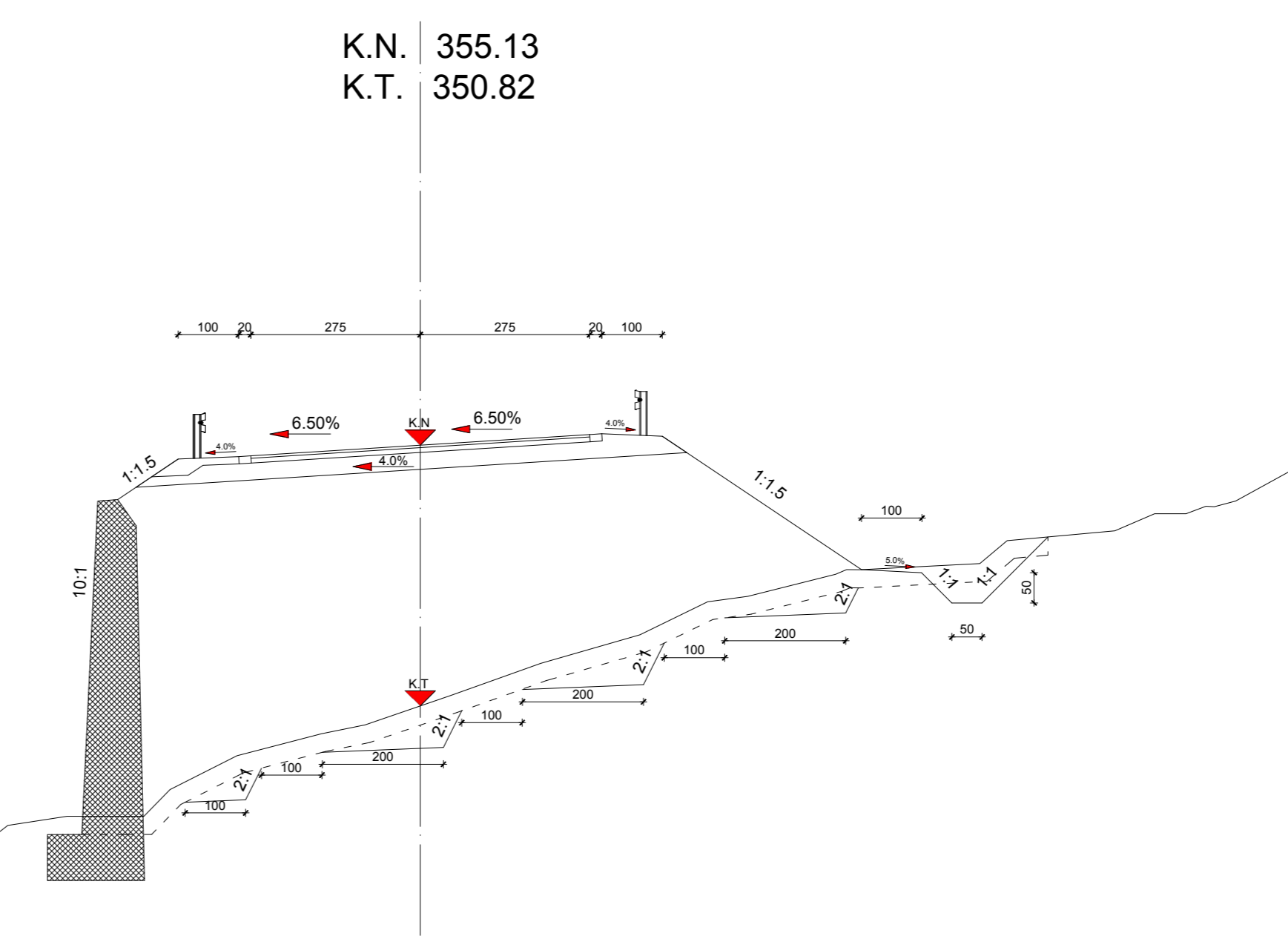
PROFIL 12 ST. 0+330.00
