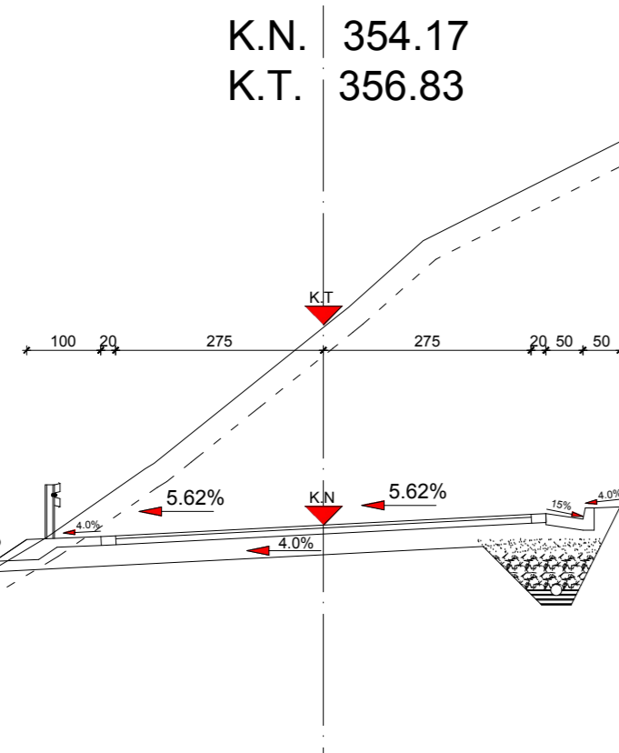
PROFIL 13 ST. 0+360.00
