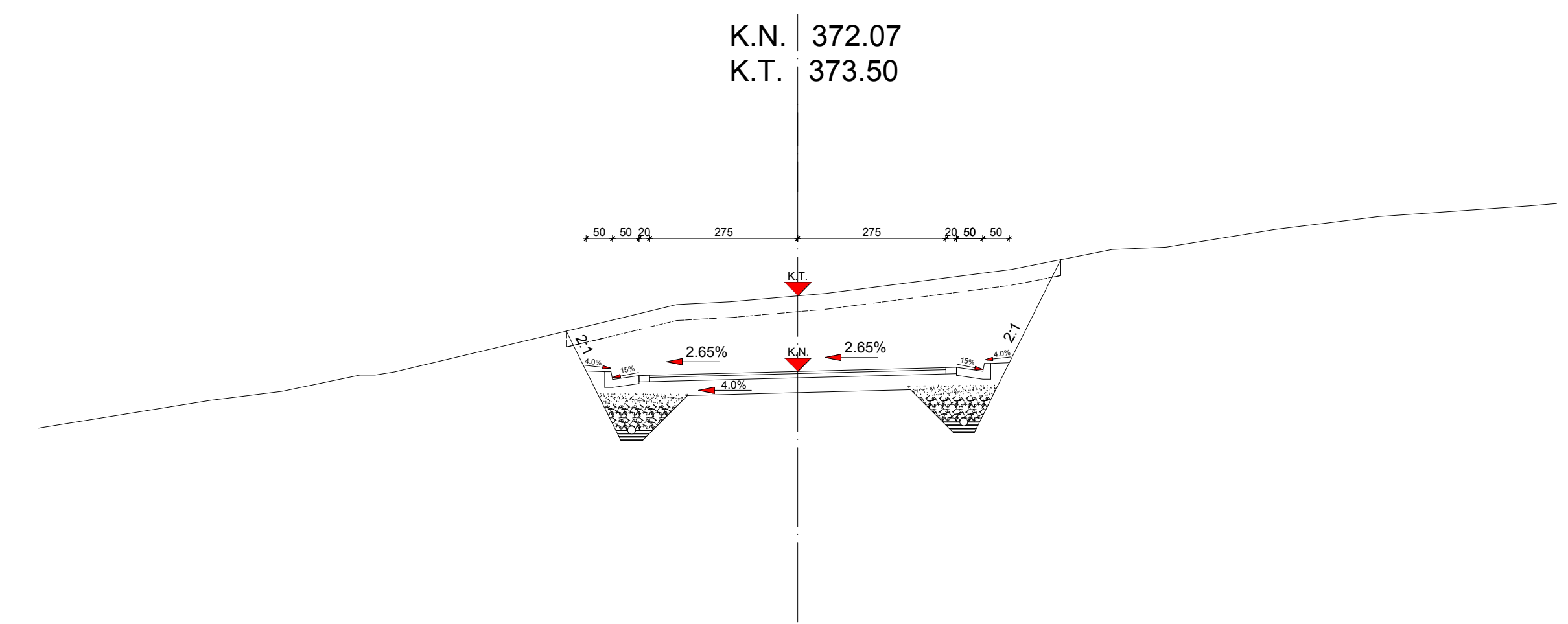
PROFIL 2 ST. 0+030.00
