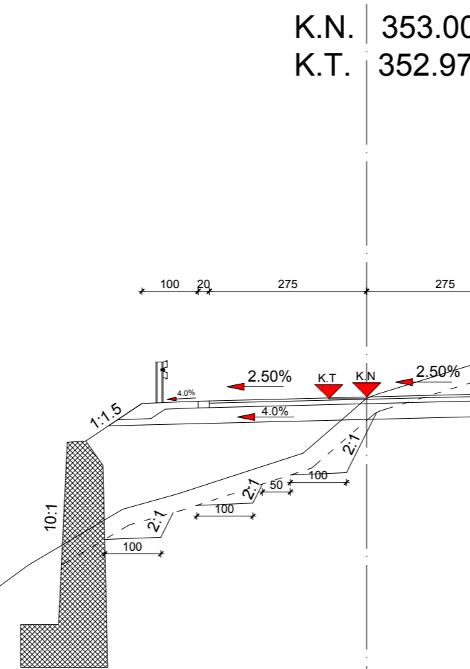
PROFIL 15 ST. 0+396.34
