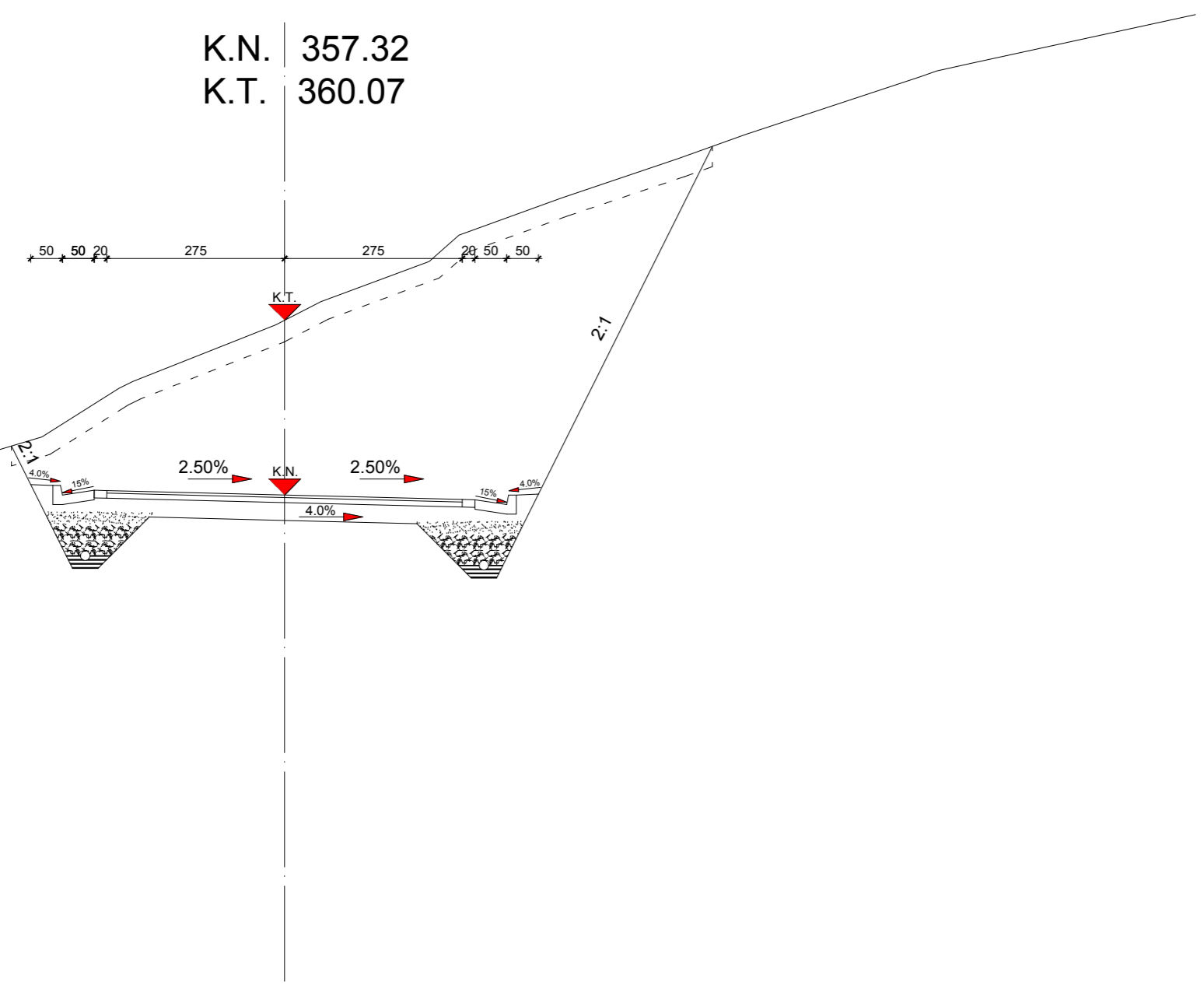
PROFIL 10 ST. 0+270.00
