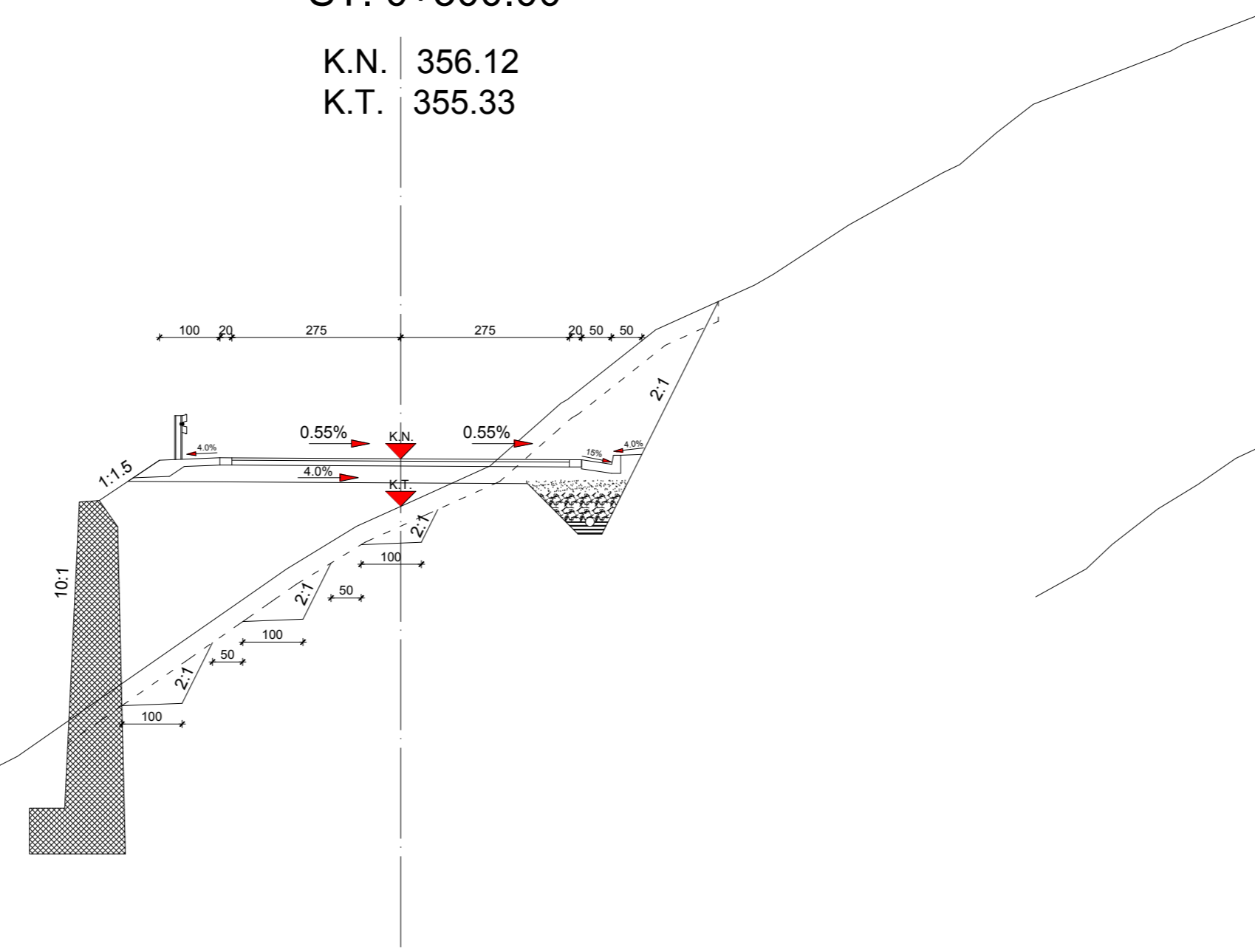
PROFIL 11 ST. 0+300.00
