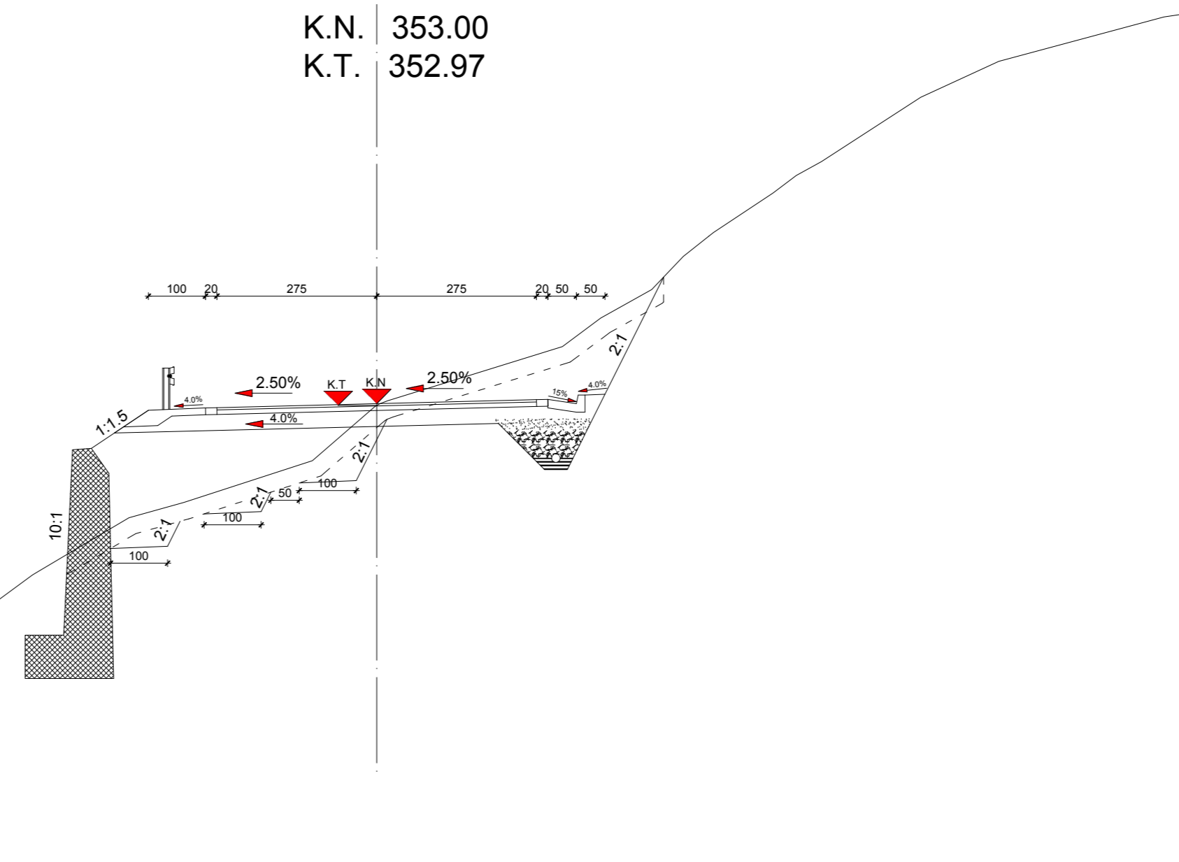
PROFIL 15 ST. 0+396.34
