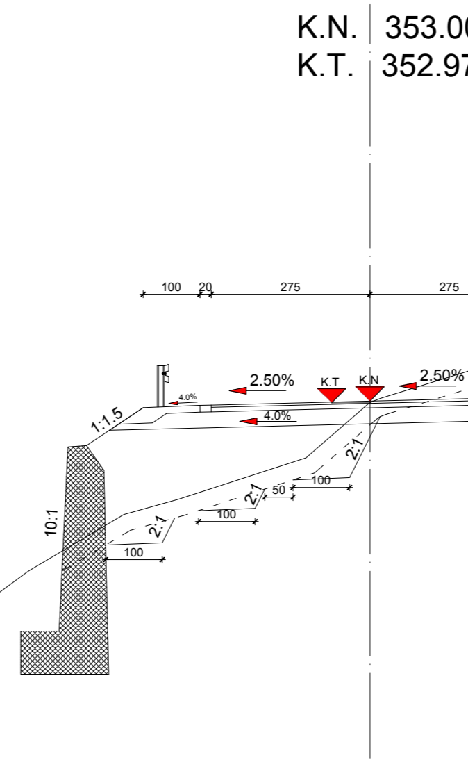
PROFIL 15 ST. 0+396.34
