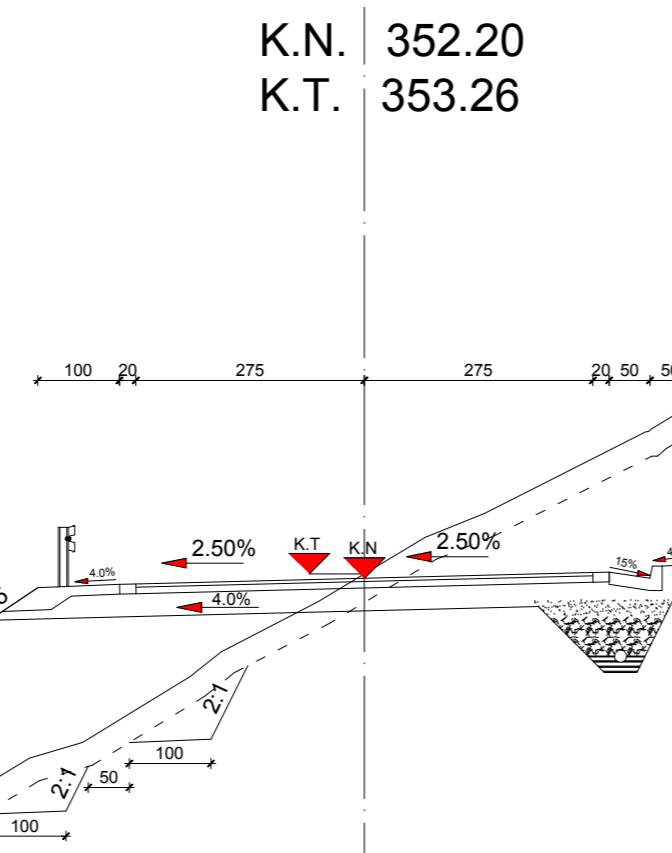
PROFIL 14 ST. 0+390.00
