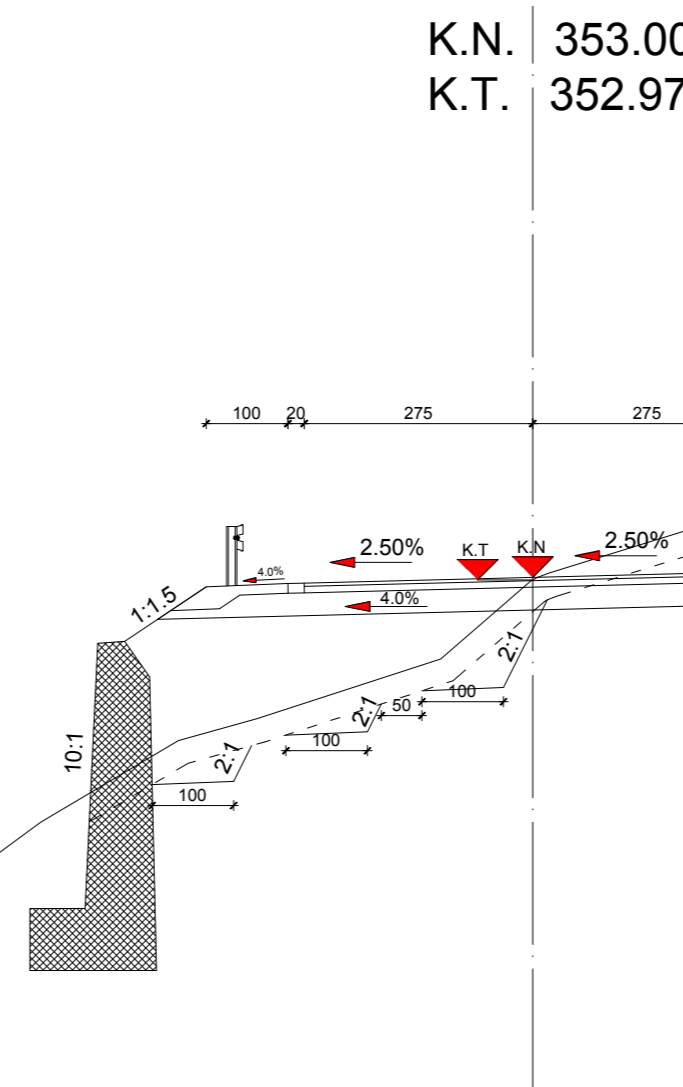
PROFIL 15 ST. 0+396.34
