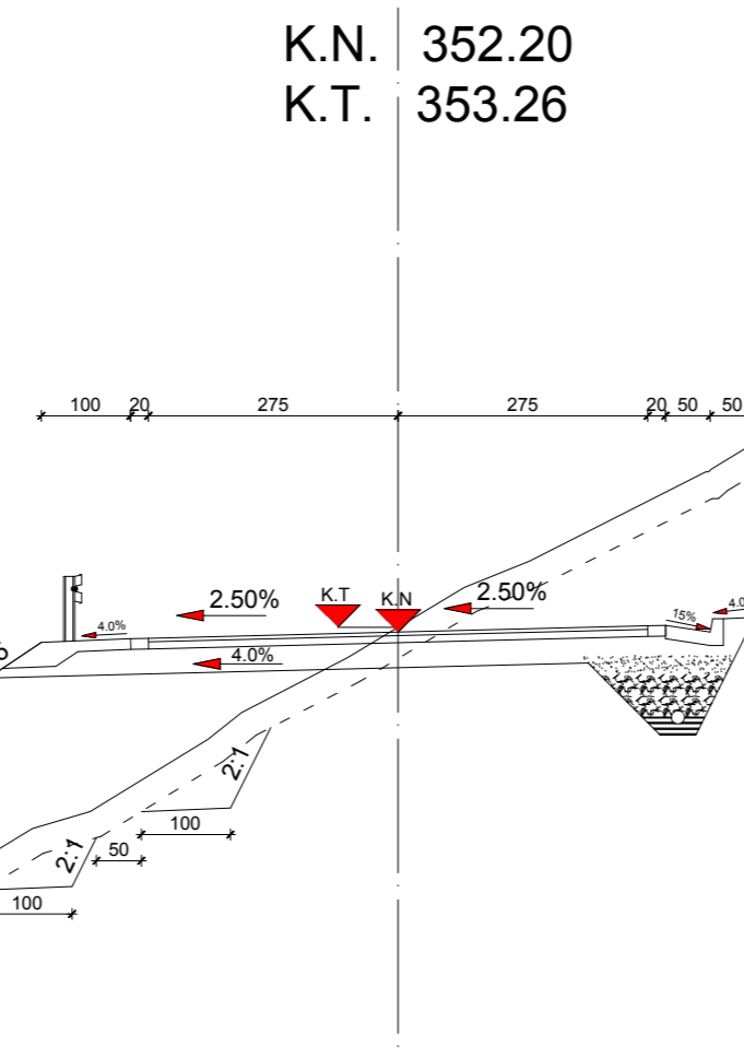
PROFIL 14 ST. 0+390.00
