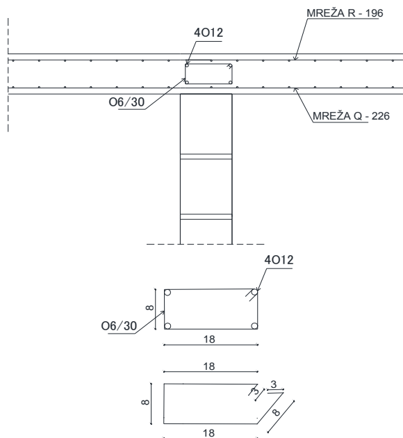
PRESJEK 2-2
