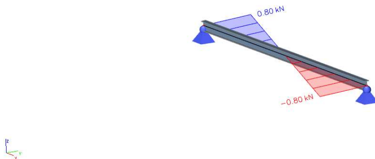
Slika 4.25. Dijagram poprečnih sila V_y za kombinaciju 1
