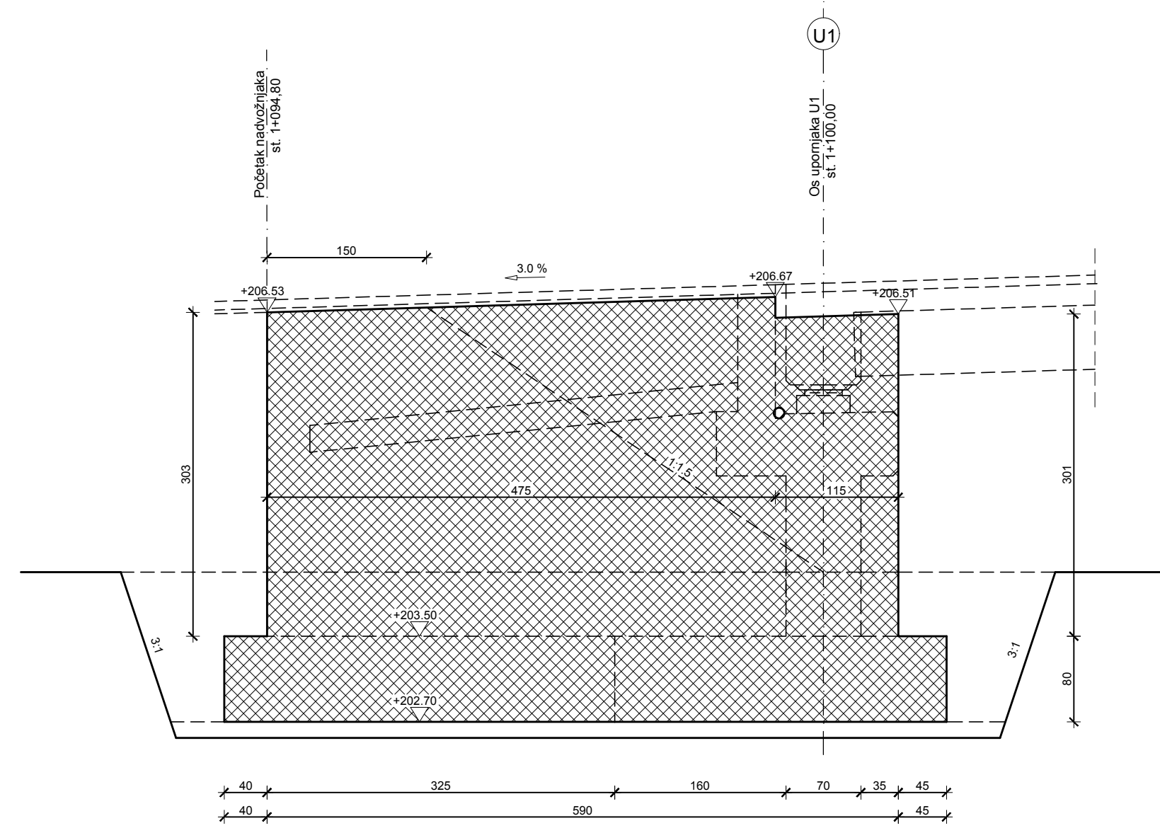
Presjek 6-6
