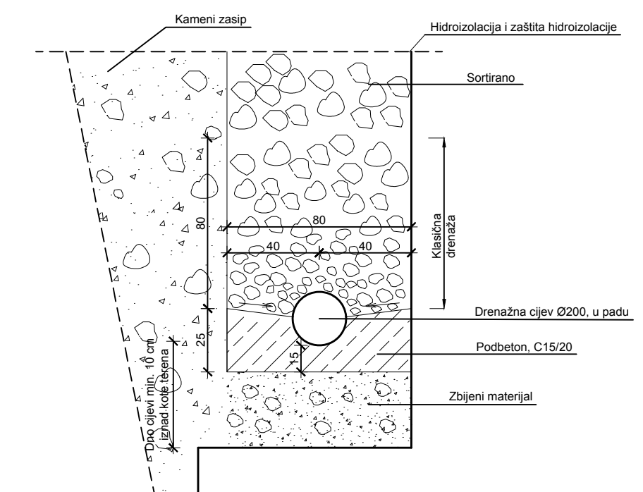
Detalj drenaze
