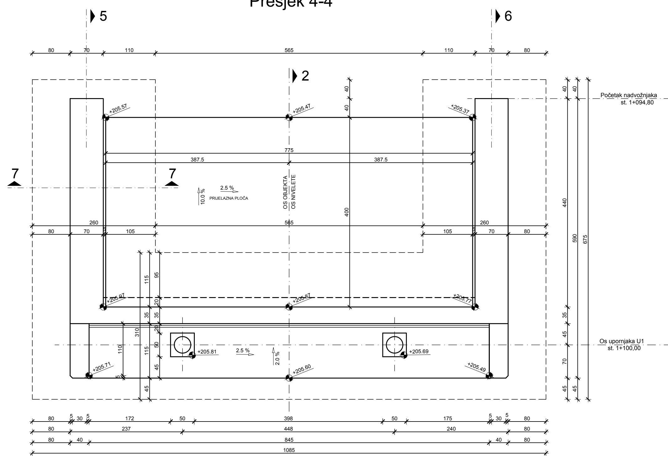
Presjek 4-4
