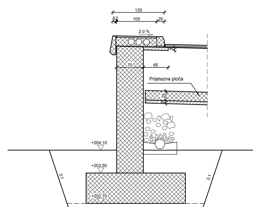
Presjek 7-7
