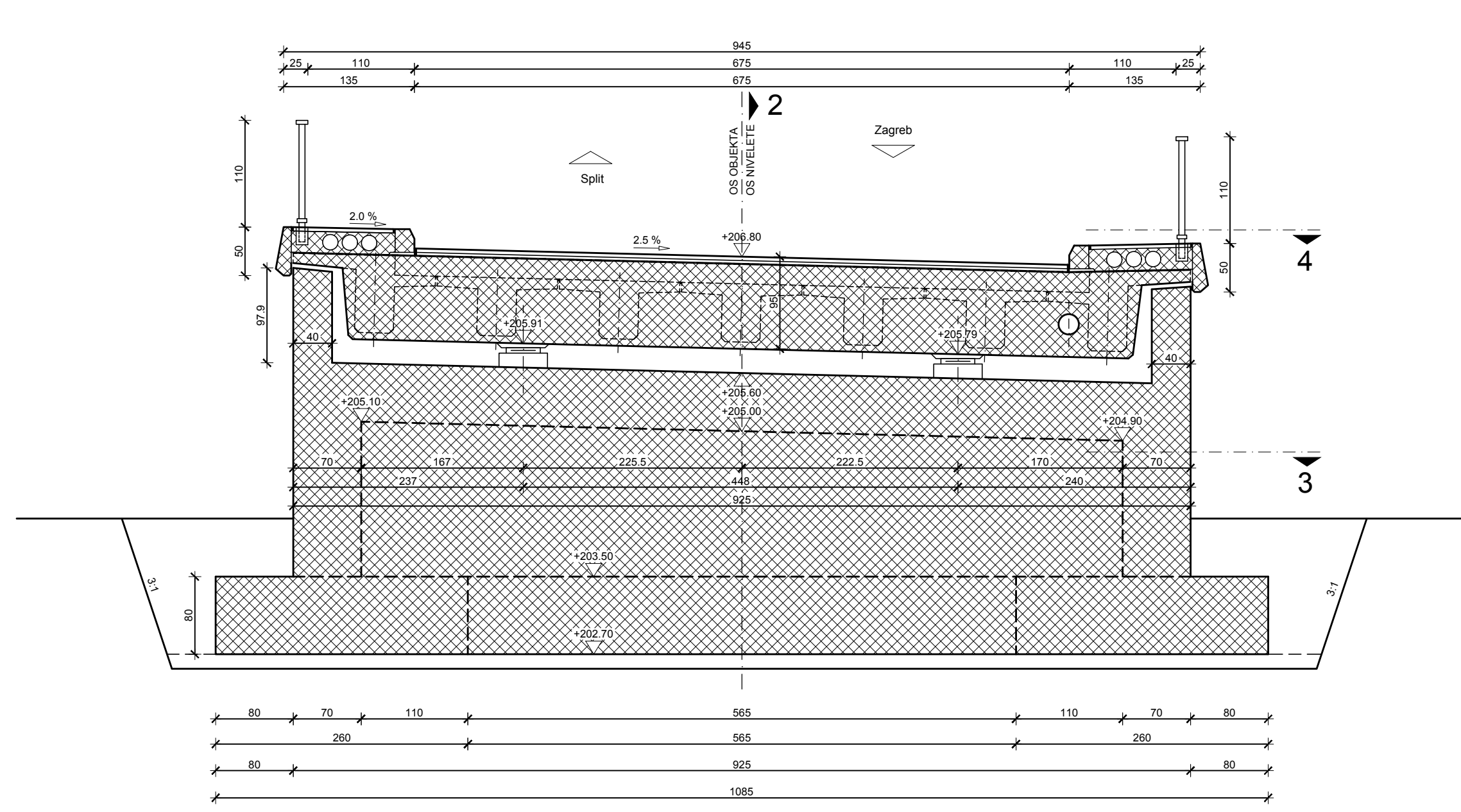
Presjek 1-1
