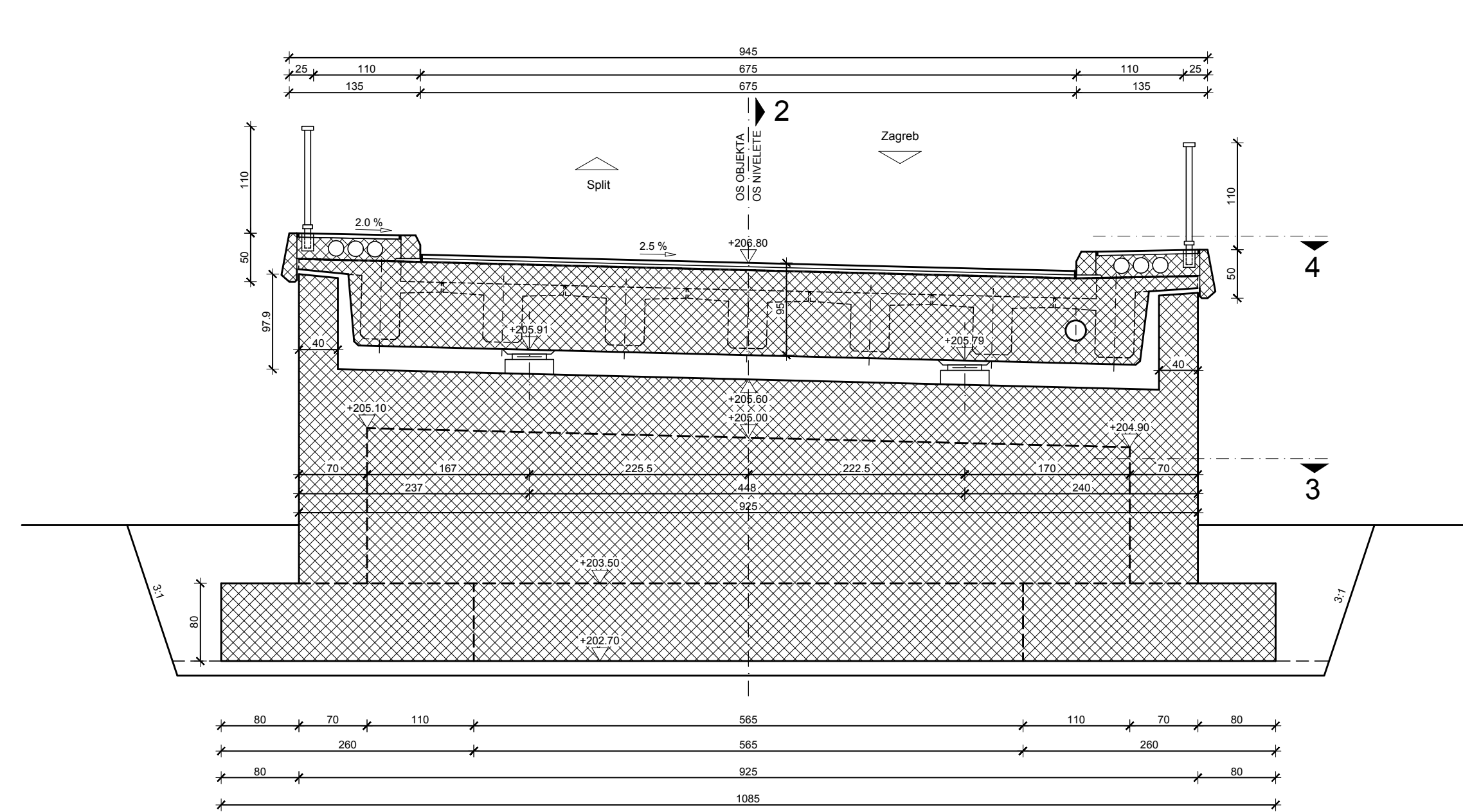
Presjek 1-1
