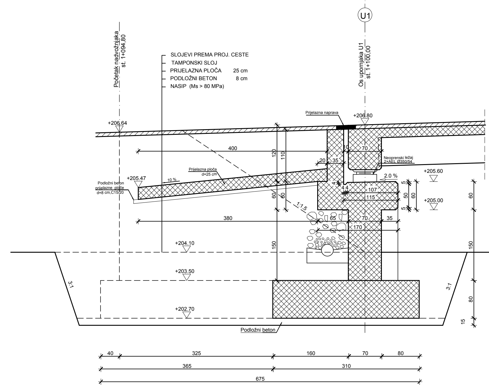
Presjek 2-2
