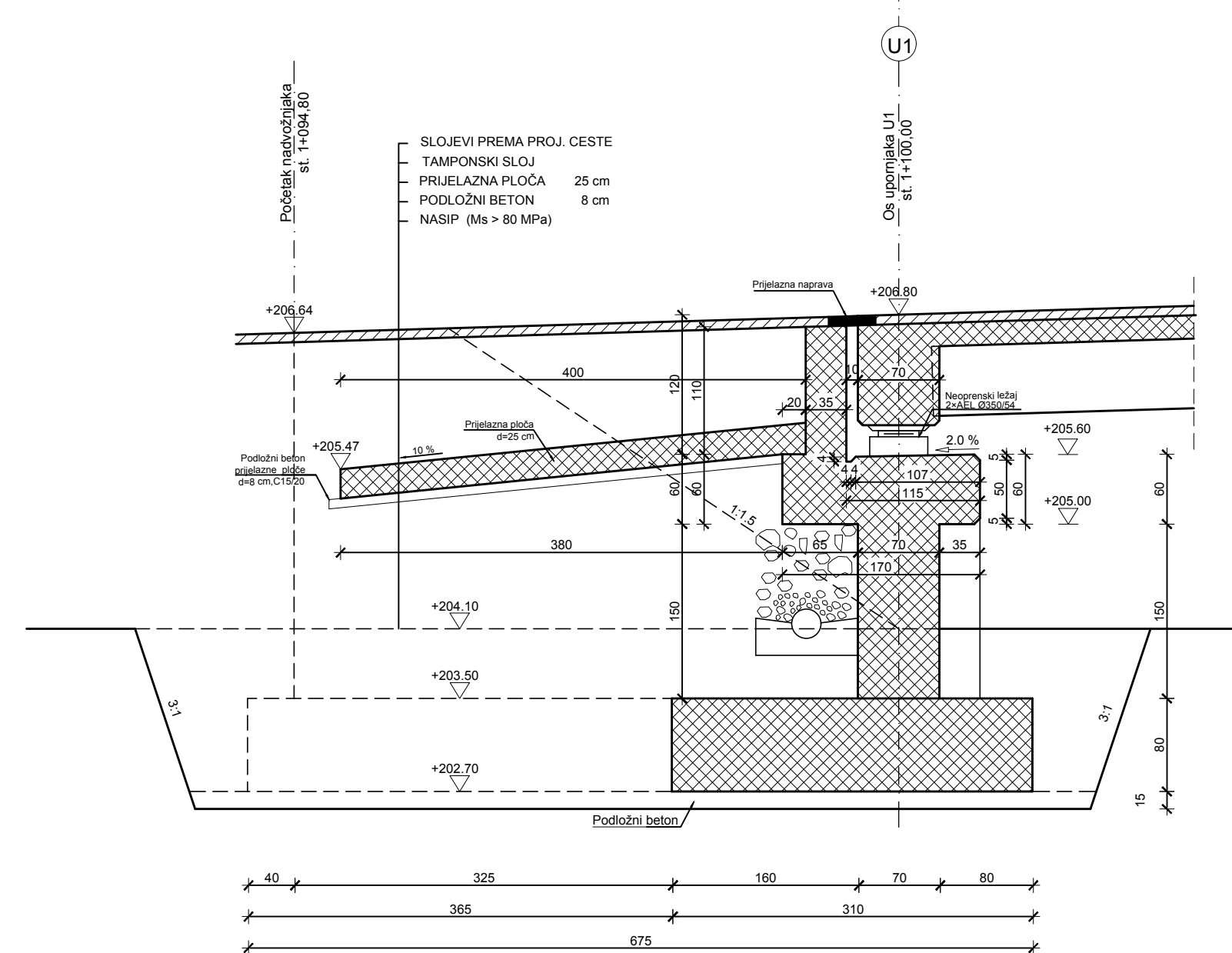
Presjek 2-2
