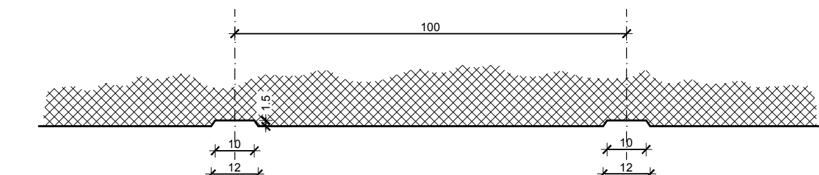
Detalj kanelura
