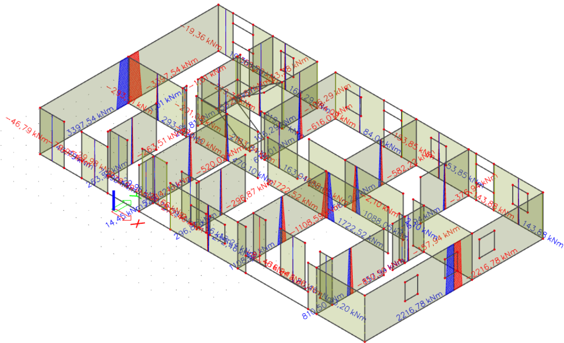
Slika 5.2: Dijagram momenata M [kN/m] za kombinaciju 1,2Sx
