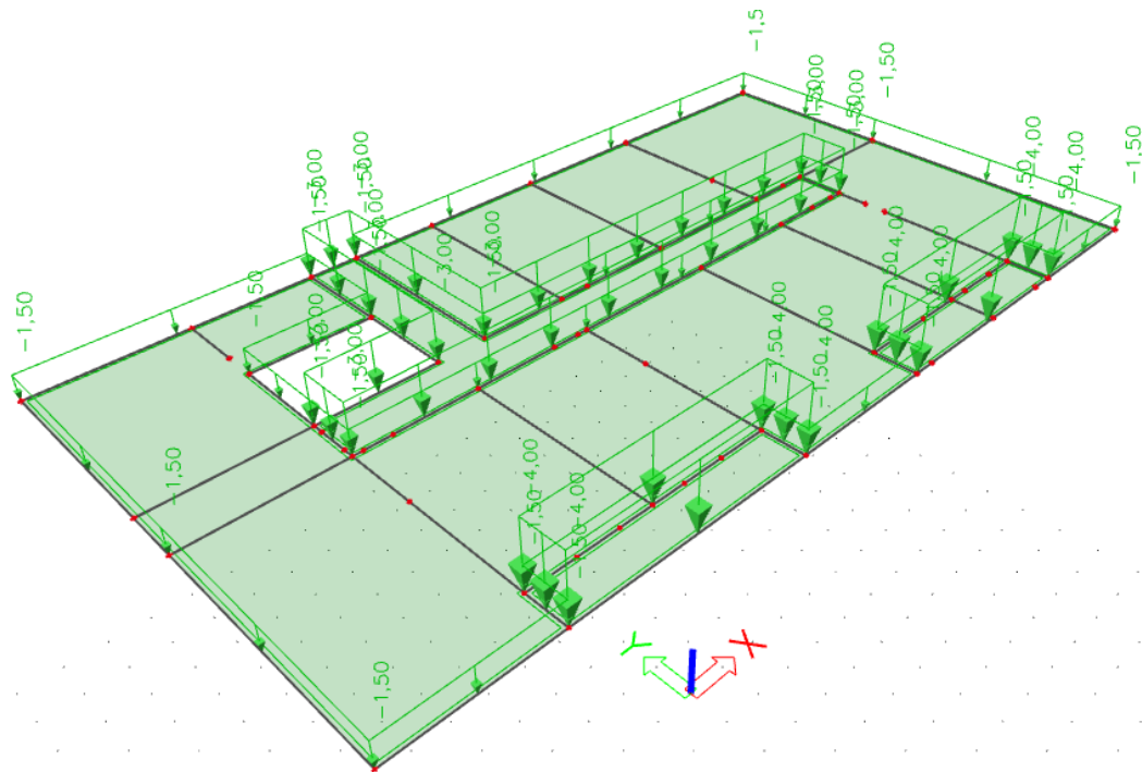
Slika 6.4: Stalno opterećenje G [ \text{kN/m}^2 ]
