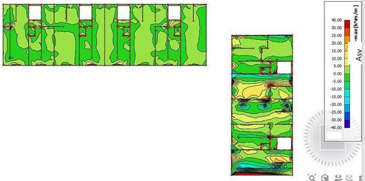
Slika 10.12. Prikaz potrebne armature A_{sy}
