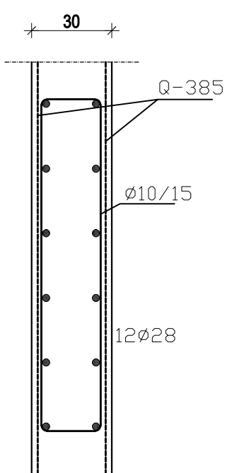
Detalj B
