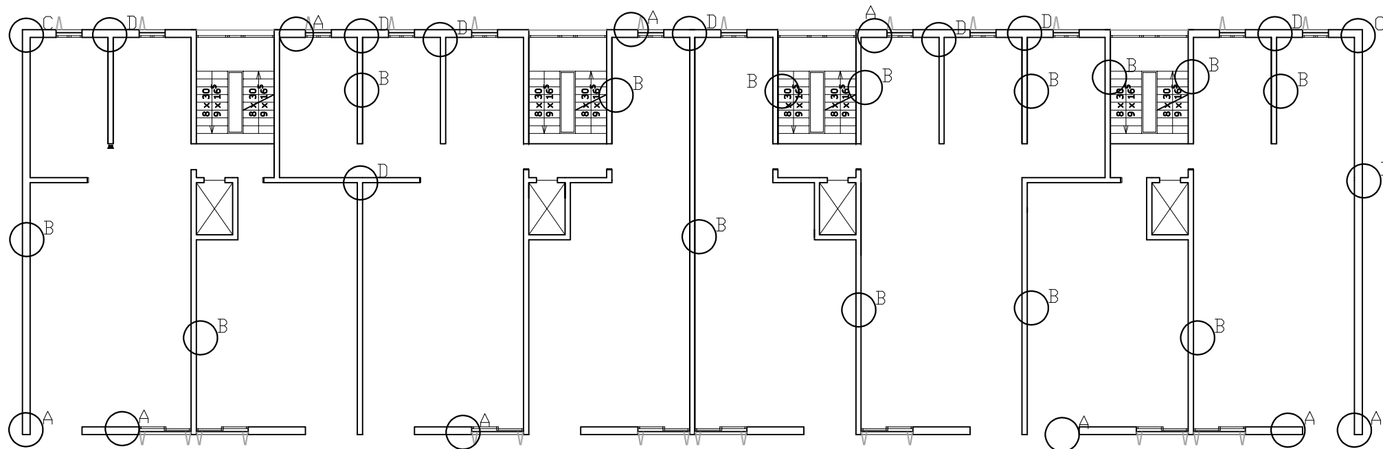
Detalj A
