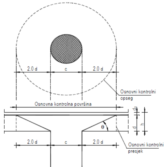
Slika 12.8. Proboj stupa kroz ploču
