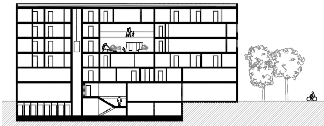
Slika 1.4. Presjek B-B
