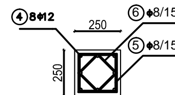
Presjek 1-1
