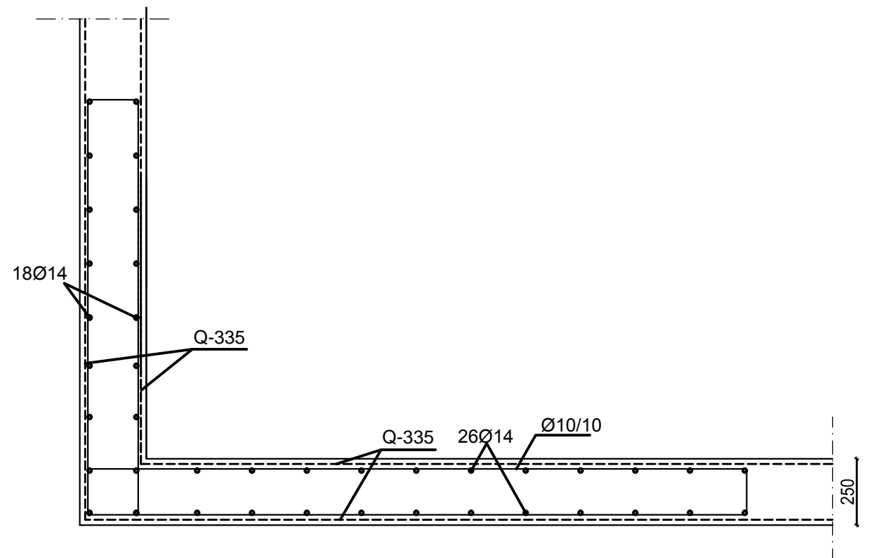
Detalj C
