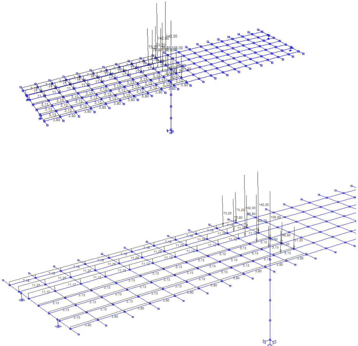
Slika 21: Pokretnno opterećenje za maksimalnu poprečnu silu pri upornjaku
