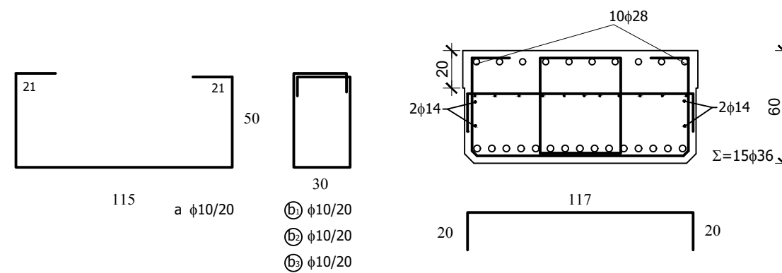
Poprečni presjek nosača(stup)
