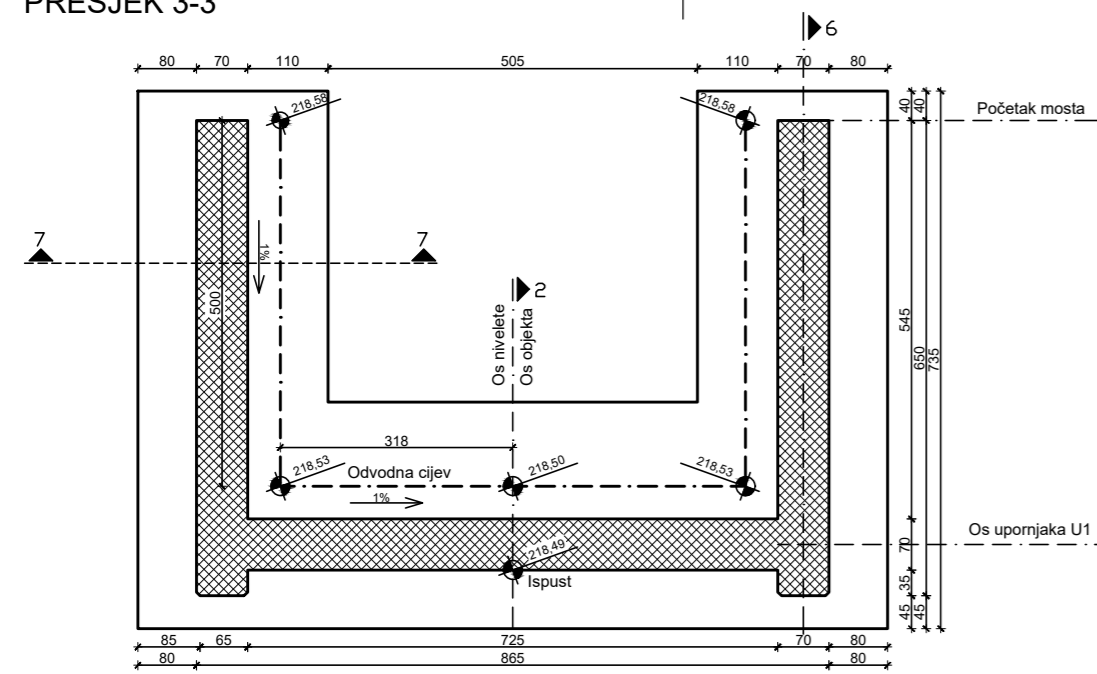
PRESJEK 3-3
