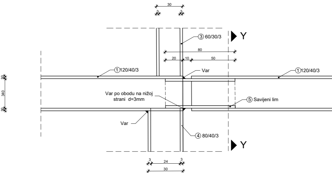
Detalj D 2 1:2
