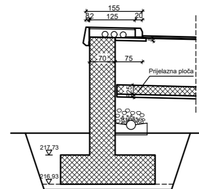
PRESJEK 7-7
