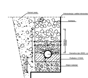
DETALJ DRENAŽE
