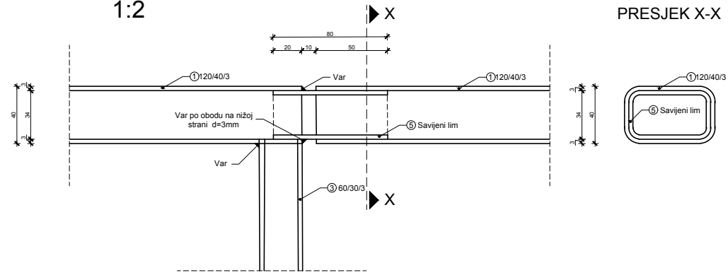
Detalj D 2 1:2
