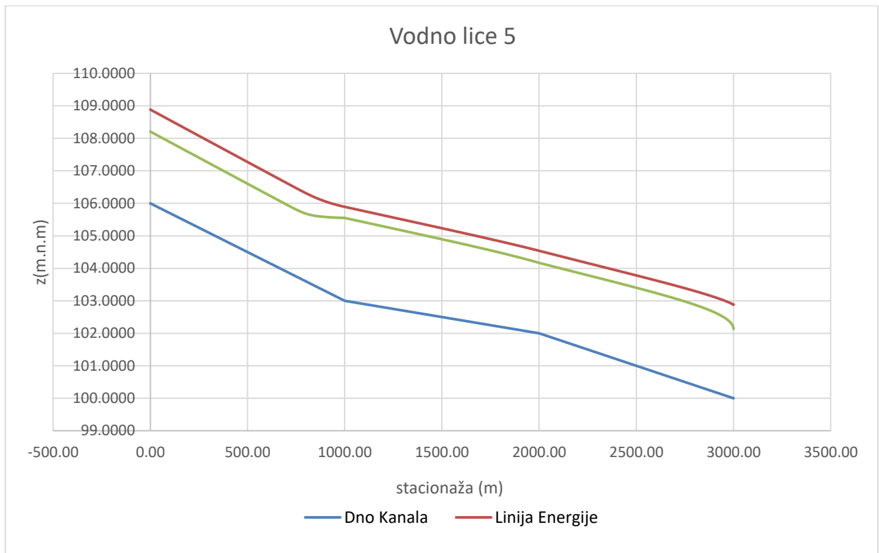
Dijagram 5. Vodno lice za protok Q_5
