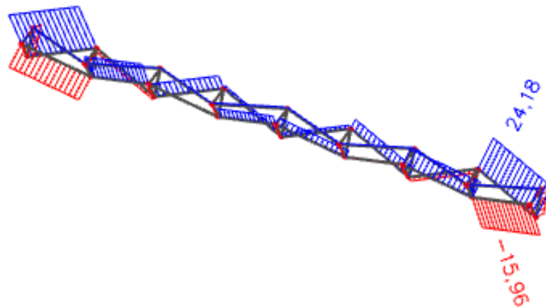
N (kN)
