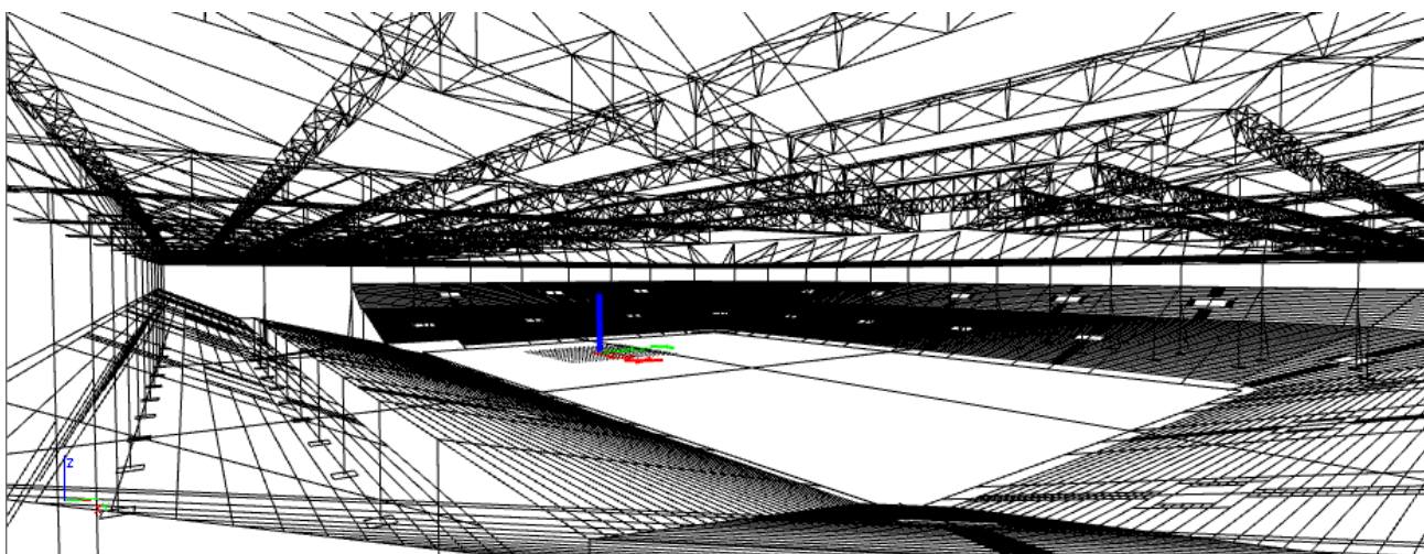
Slika 8.26: Perspektiva pogled s unutarnje strane sjeverozistok
