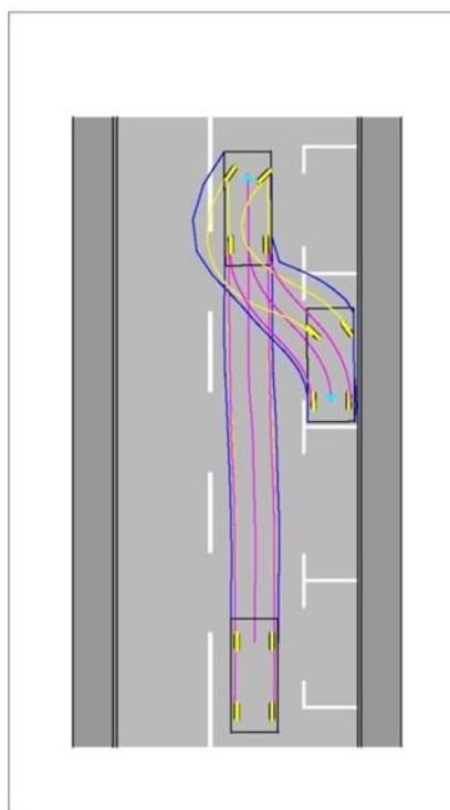
Slika 12 Manevar potreban za uspješno uzdužno parkiranje [2]
