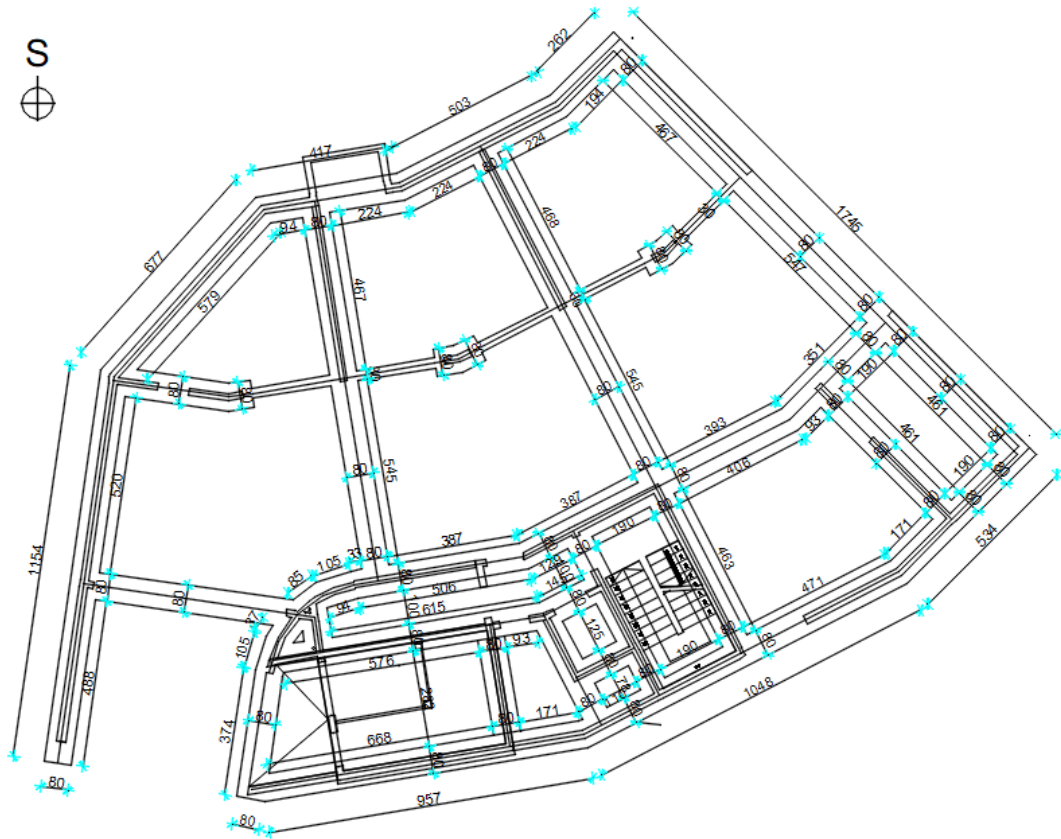
Slika 1.6. Tlocrt temelja
