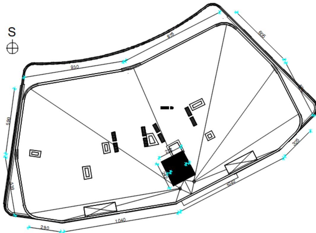
Slika 1.12. Tlocrt krova
