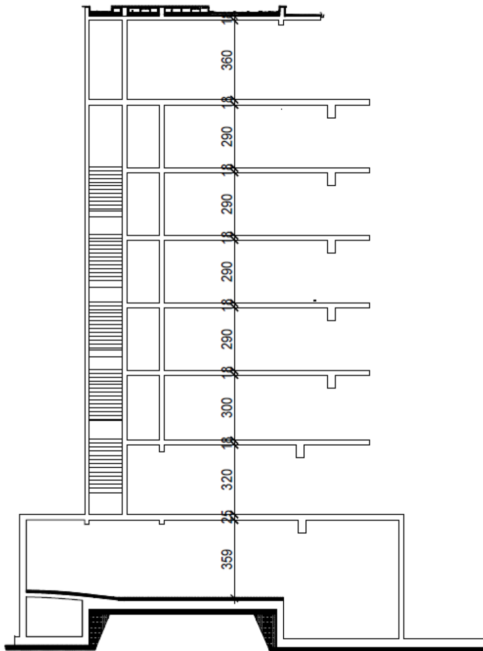
Slika 1.16 Karakteristični presjek B-B
