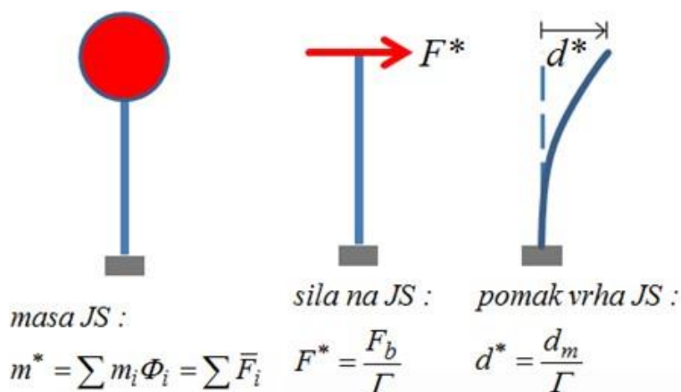
Slika 6.8: Prikaz ekvivalentnog jednostupnjevno sustava sa silom F^* i pomakom d^*
