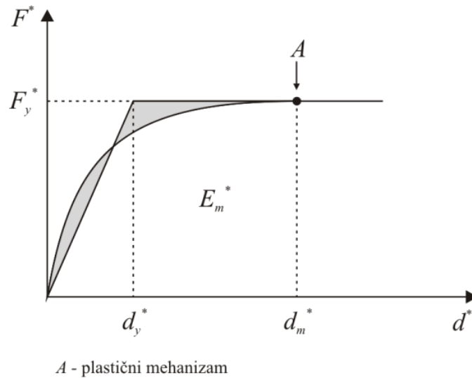
Slika 6.9: Određivanje idealnog elasto-plastičnog dijagrama
