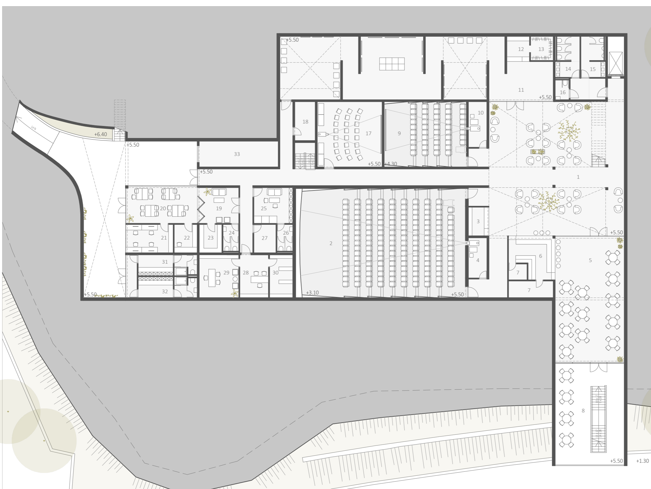
TLOCRT PODRUMA
