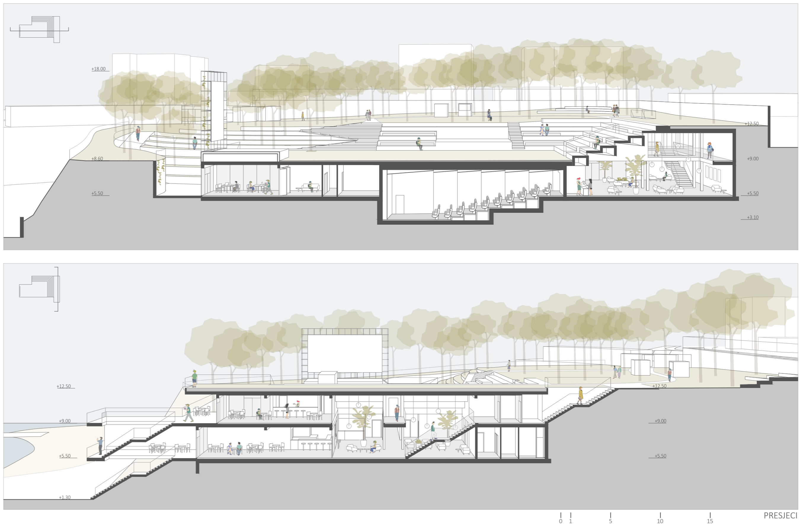
0 1 5 10 15 PRESJECI
