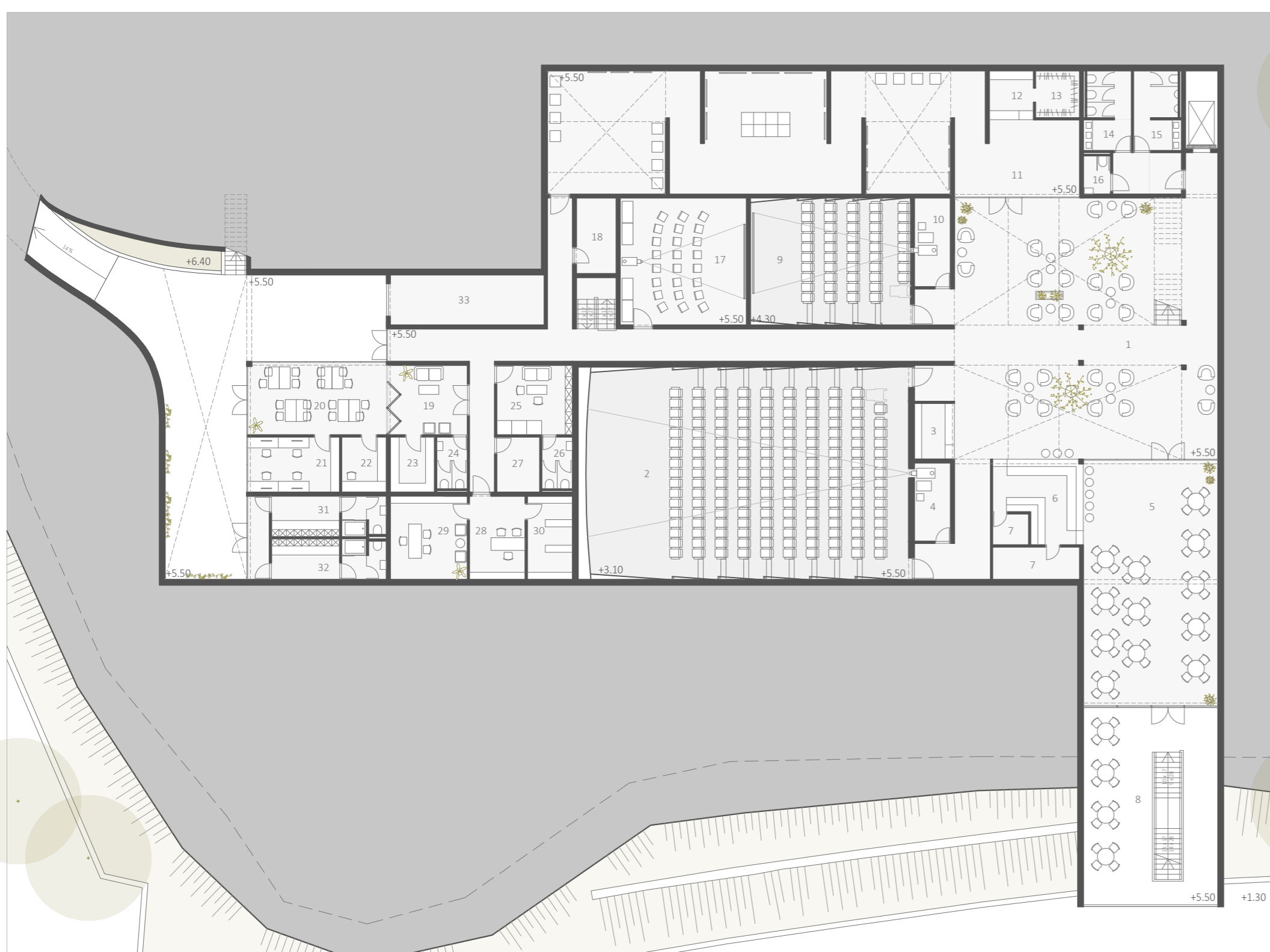
TLOCRT PODRUMA
