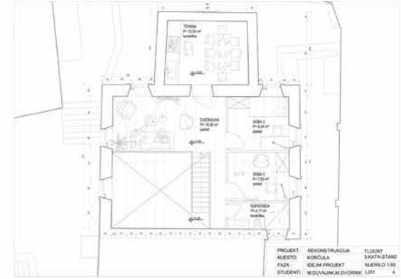
PROJEKT REKONSTRUKCIJA TLOCRT Mjesto: KORČULA 2. KATA-STANJ FAZA: IDEJN. PROJEKT Mjersko 1:50 STUDENTI: M. DUJANIĆ I M. DVORNIK LIST 3
