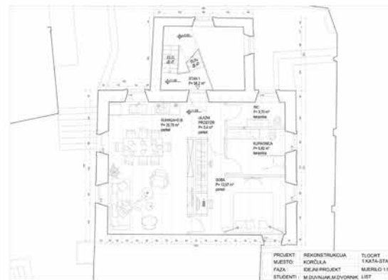
PROJEKT REKONSTRUKCIJA TLOCRT POD- Mjesto KORUČULA PROZEMALJA Faza IDEJN PROJEKT Mjersko 1:50 Studenti: M.DUNJAK I M.DVORNİK LIST 1
