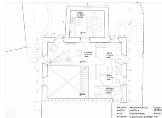
PROJEKT REKONSTRUKCIJA TLOCRT Mjesto KORUČULA 2. KATA Faza IDEJN PROJEKT Mjersko 1:50 Studenti: M.DUNJAK I M.DVORNİK LIST 3
