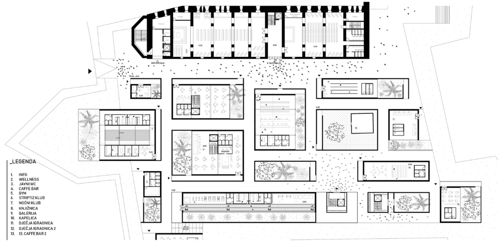
TLOCRT PRIZEMLJA
