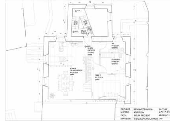
PROJEKT REKONSTRUKCIJA TLOCRT Mjesto: KORČULA I KATA-STANJ Faza: IDEJN PROJEKT Mjersko 1:50 Studenti: M.DUJANJAK I M.DVORNİK LIST 2
