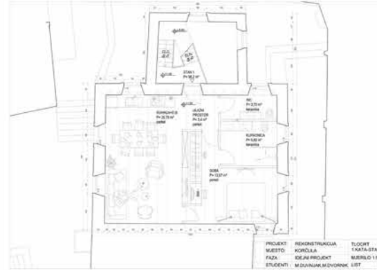
PROJEKT REKONSTRUKCIJA TLOCRT POB. Mjesto: KORČULA PROJEKCIJA Faza: IDEJN PROJEKT Mjersko 1:50 Studenti: M.DUJANJAK I M.DVORNİK LIST 1
