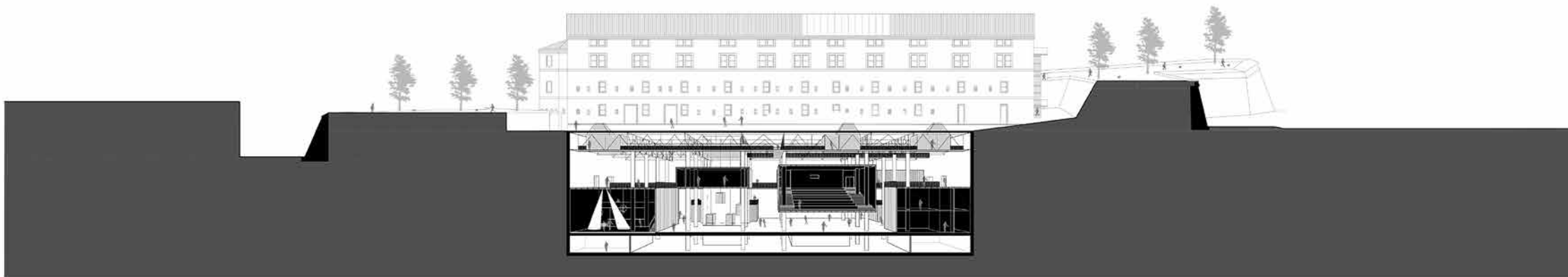
PRESJEK U PERSPEKTIVI
