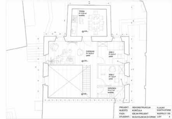
PROJEKT REKONSTRUKCIJA TLOCRT Mjesto: KORČULA I KATA-STANJ Faza: IDEJN PROJEKT Mjersko 1:50 Studenti: M.DUJANJAK I M.DVORNİK LIST 3
