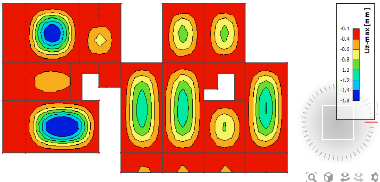
Slika 8.29. Prikaz progiba
