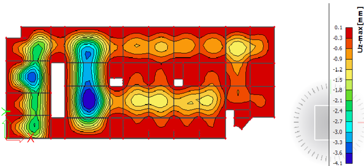
Slika 8.71. Prikaz progiba
