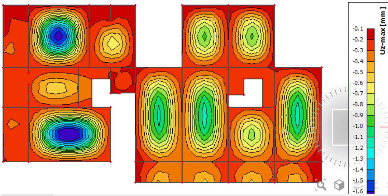
Slika 8.22. Prikaz progiba
