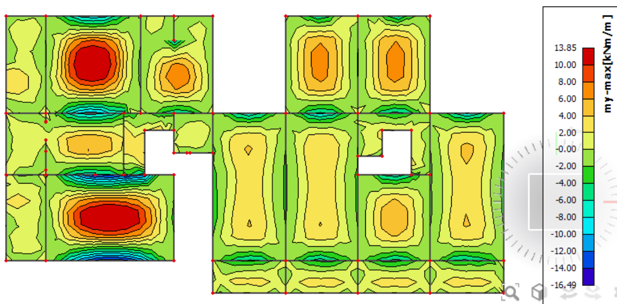
Slika. 8.18. M_y
