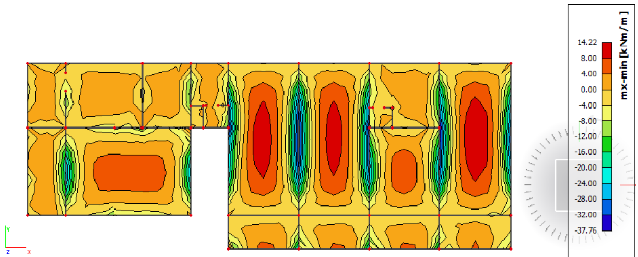
Slika 8.4. M_x
