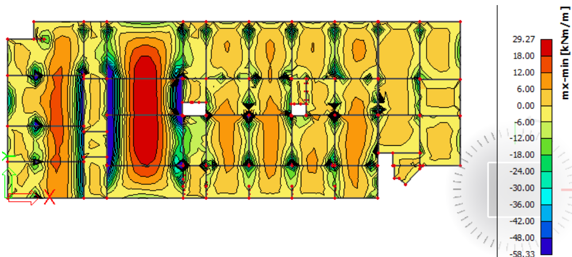
Slika 8.76. M_x
