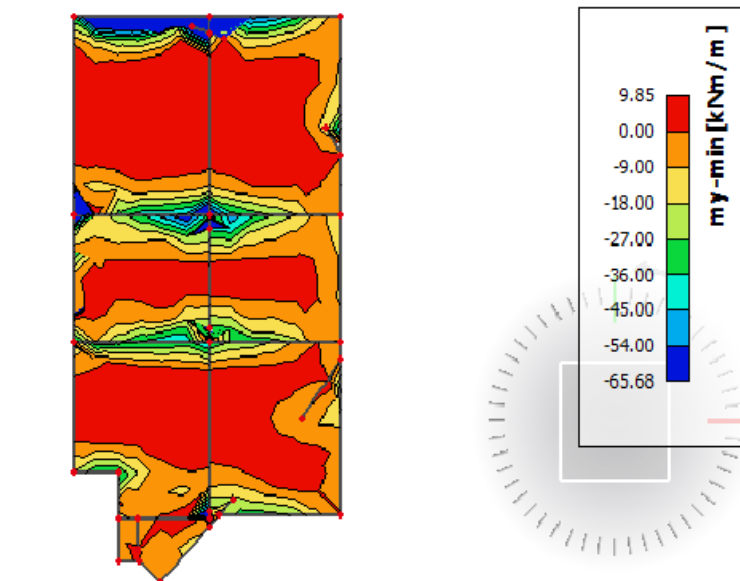
Slika 8.62. M_y
