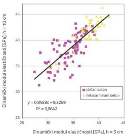
Slika 4.25. Regresijski pravac uzoraka visine 5 i 10cm ( R = 0,81 ) [9]
