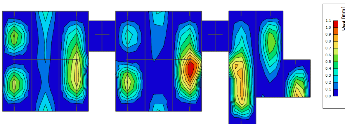
Slika 11.92 Prikaz progiba - GSU
