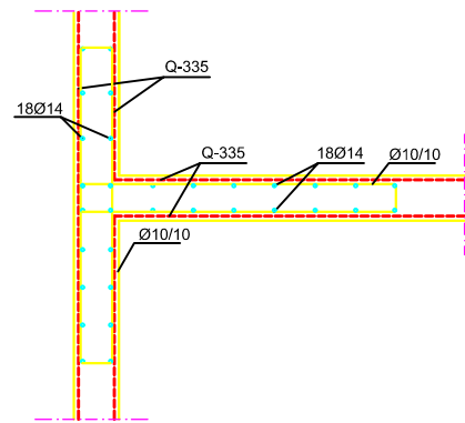
Detalj A
