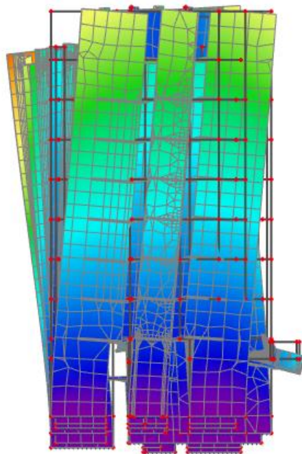
Slika 10.8 Drugi vlastiti vektor od djelovanja potresa na konstrukciju
