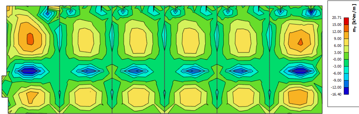
Slika 11.30 Prikaz momenata savijanja - m_y
