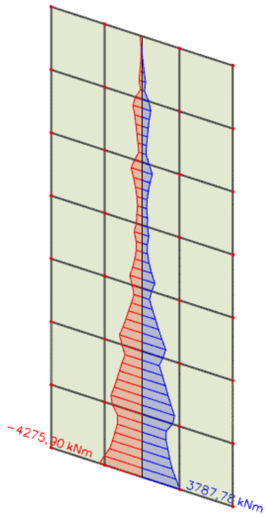
Slika 13.8 Moment savijanja M
