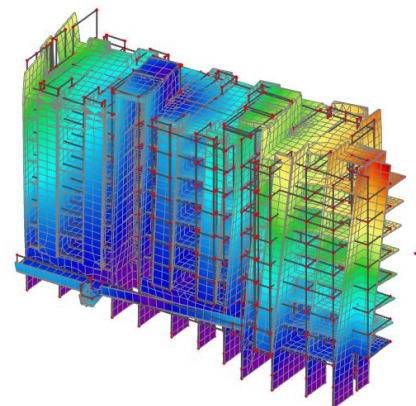
Slika 10.8 Drugi vlastiti vektor od djelovanja potresa na konstrukciju
