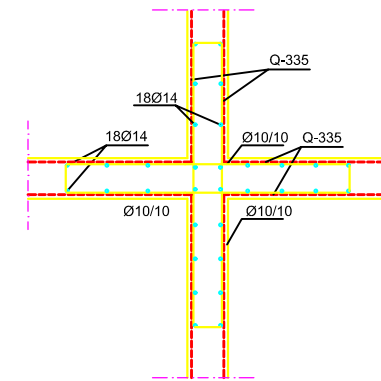
Detalj E
