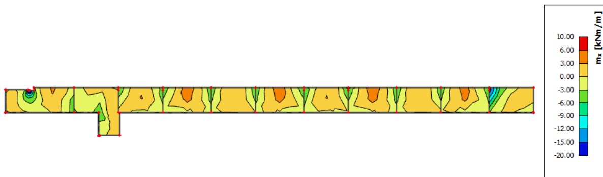
Slika 11.47 Maksimalni momenti savijanja – GSU
