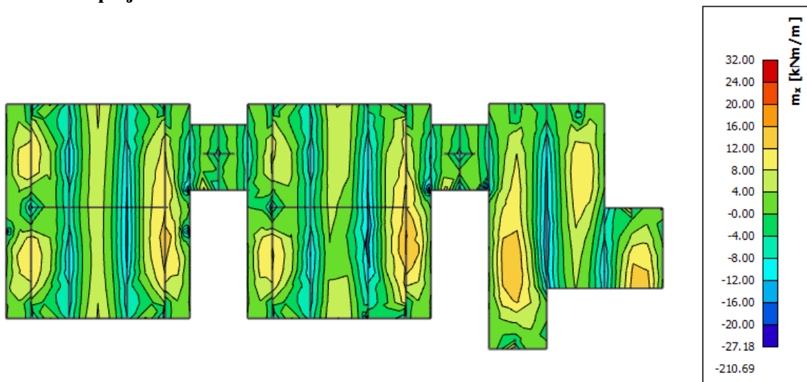
Slika 11.87 Prikaz momenata savijanja – m_x
