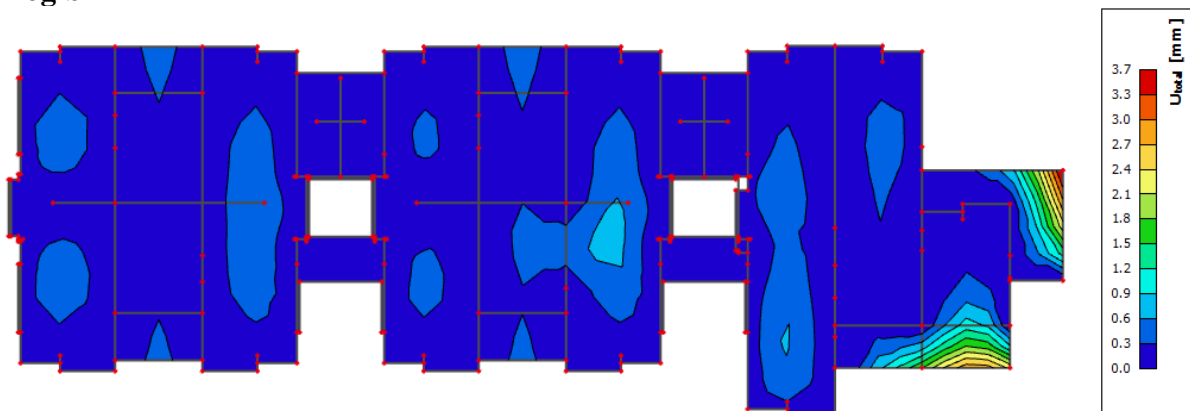
Slika 11.84 Prikaz progiba - GSU
