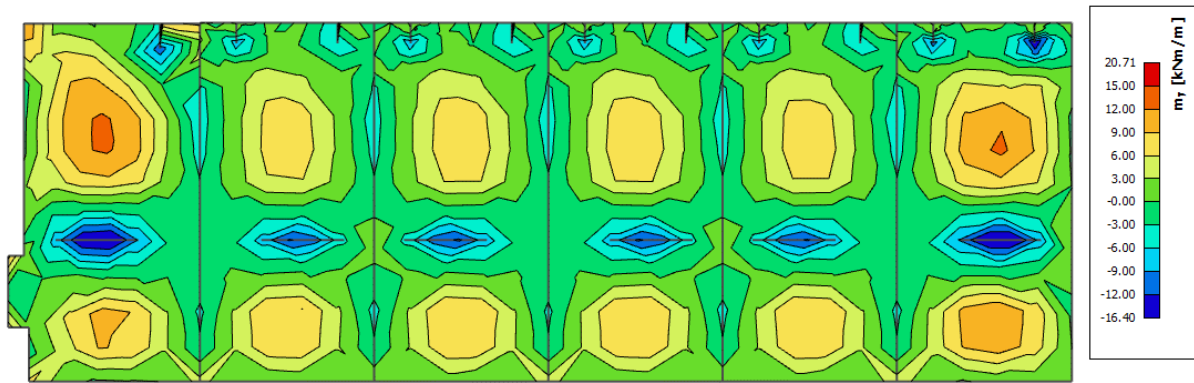
Slika 11.30 Prikaz momenata savijanja - m_y
