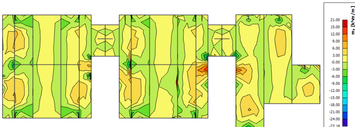
Slika 11.88 Prikaz momenata savijanja - my
