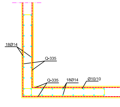
Detalj B
