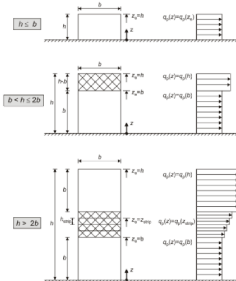
Slika 8.10 Referentna visina z_e u ovisnosti o h i b , te odgovarajući profil brzina
