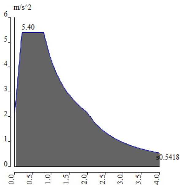
Slika 30 Proračunski spektralni ubrzanja za unesene podatke
