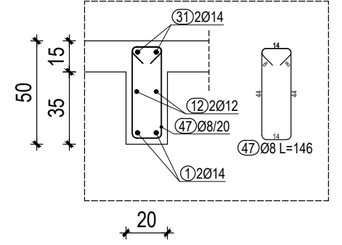
DETALJ 1-1 M 1:25
