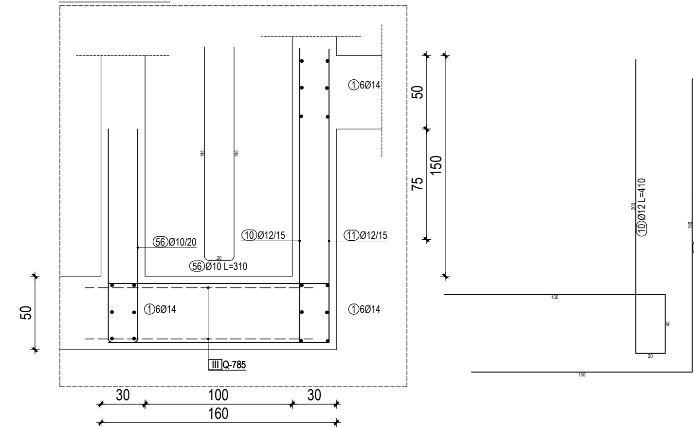
DETALJ 2-2 M 1:25
