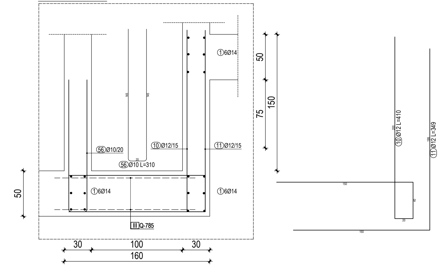
DETALJ 2-2 M 1:25
