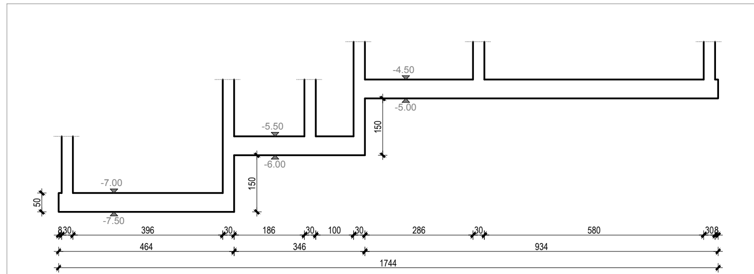
PRESJEK 1-1
