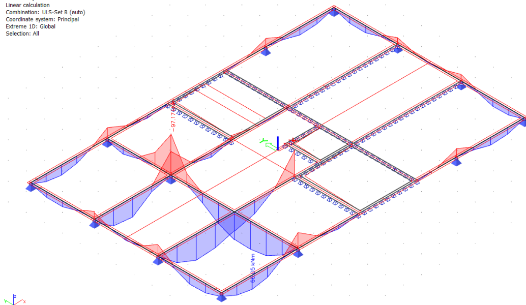
Slika 70 Dijagram momenta savijanja na gredama M_y
