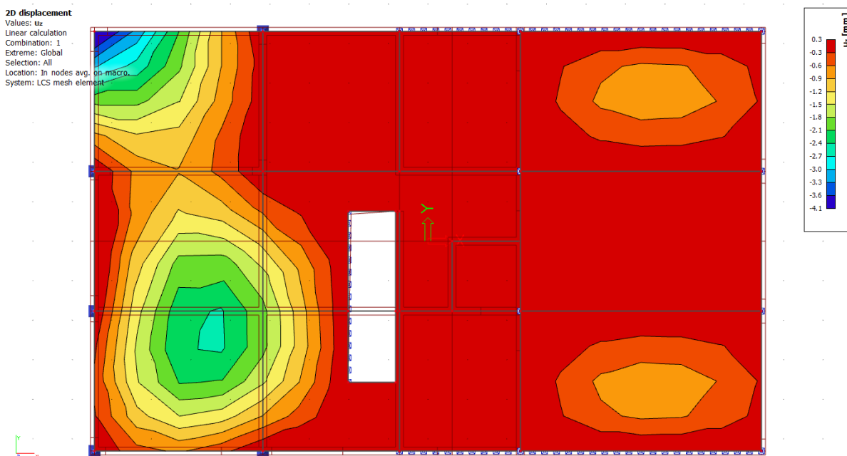
Slika 77 Vrijednost progiba na ploči
