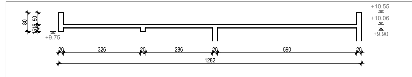
PRESJEK 1-1
