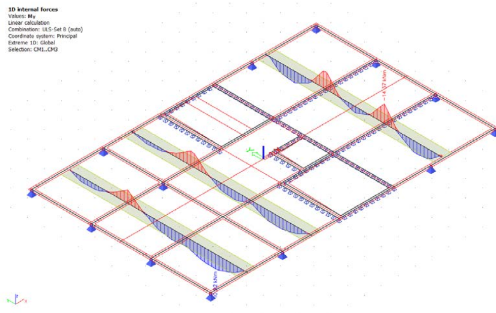
Slika 64 1D dijagram momenata savijanja m_y (duži smijer)
