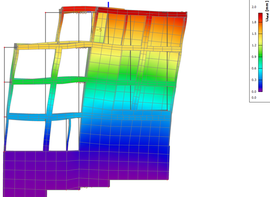
Slika 40 Translacija u smjeru globalne osi X (1)
