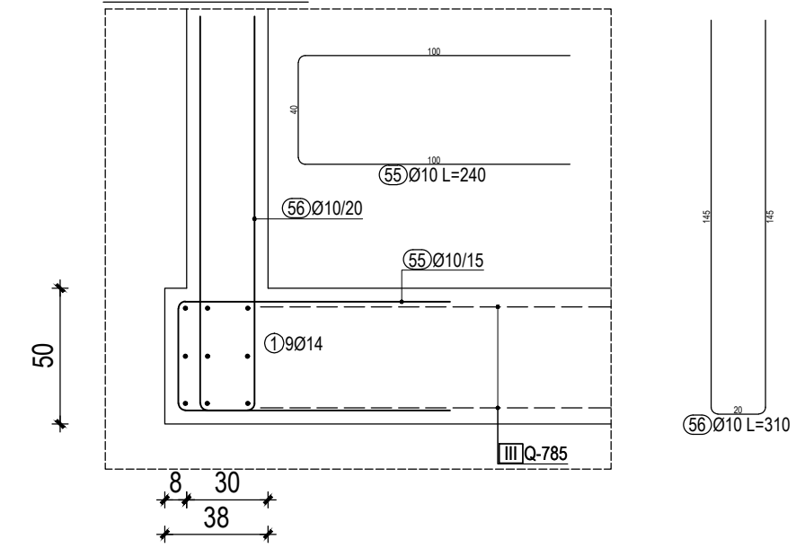
DETALJ 2-2 M 1:25
