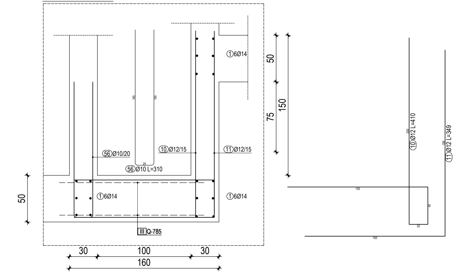
DETALJ 2-2 M 1:25
