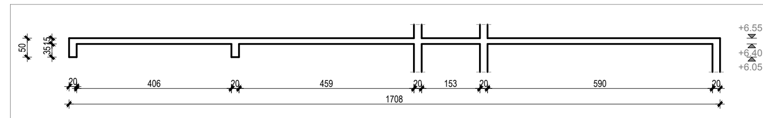
PRESJEK 1-1
