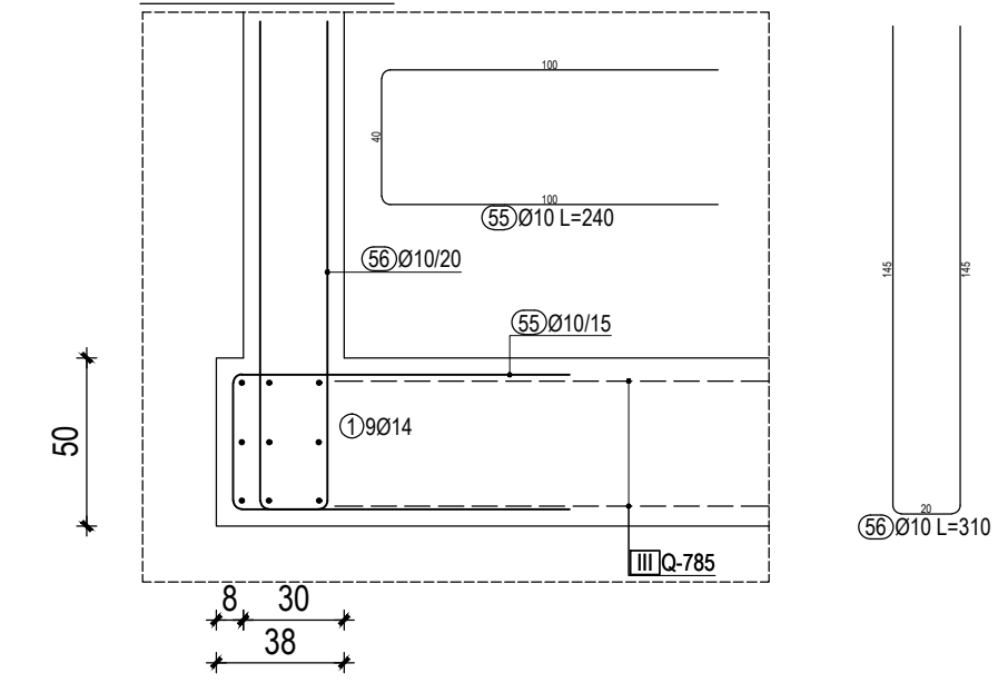
DETALJ 2-2 M 1:25
