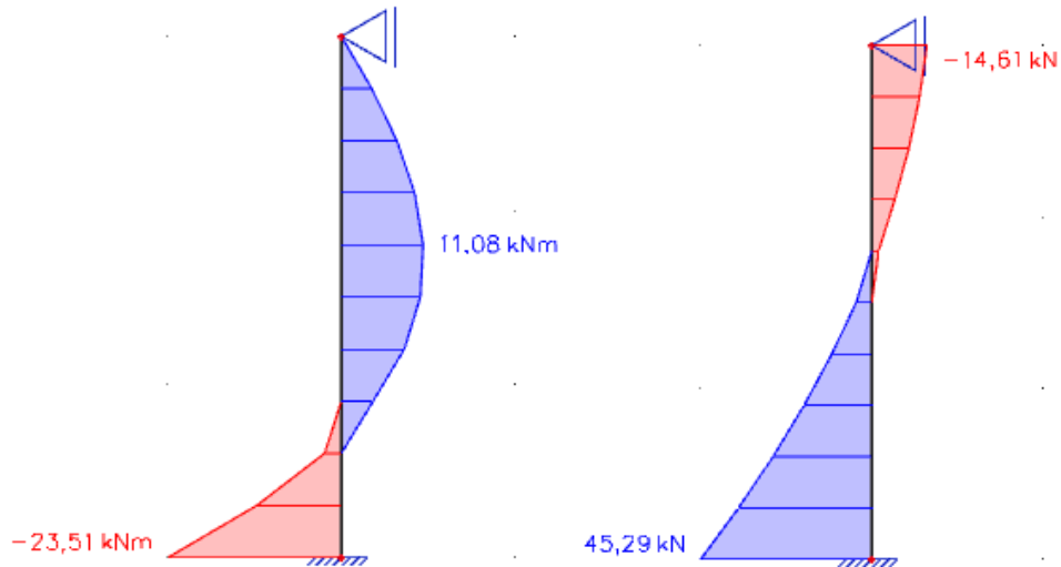
Slika 10.2. Prikaz momenata savijanja M_y i poprečnih sila V_z za mjerodavnu kombinaciju
