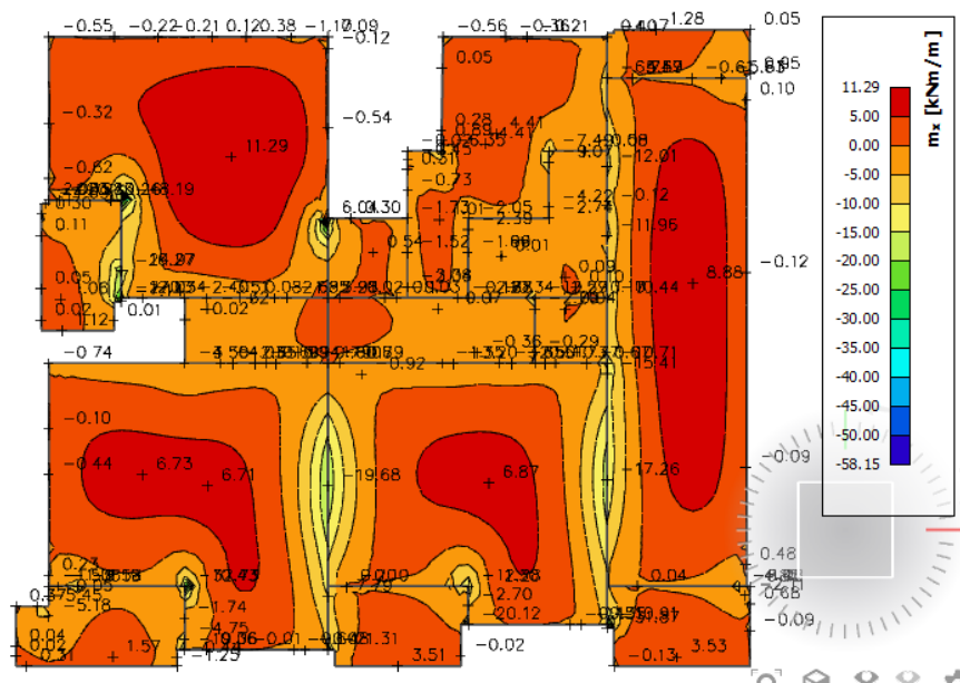
Slika 5.5. Moment savijanja M_{Ed,x} ( \text{kNm/m} ) za GSU-1
