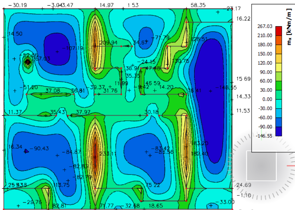
Slika 12.6. Momenti savijanja M_{sd,x} [kNm/m] za GSN-1
