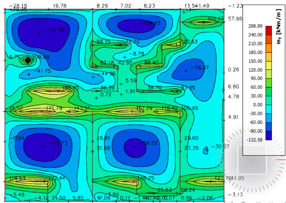
Slika 12.7. Momenti savijanja M_{sd,y} [kNm/m] za GSN-1
